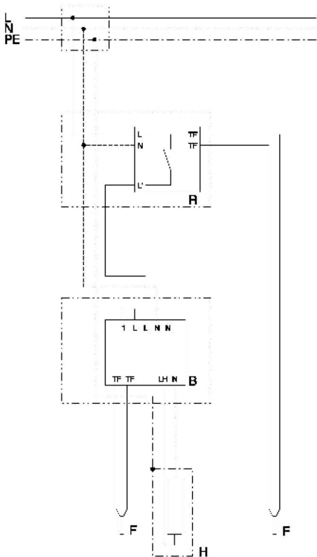
Принципиальная схема
