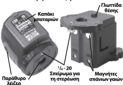
Εικόνα 3 - Μέρη του αλφαδιού λέιζερ
