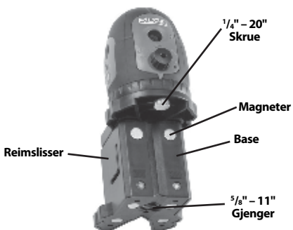
Fig. 6 – Base
