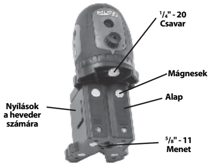
6. ábra - Alapzat
