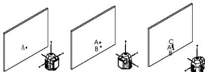
Figura 9 - Autocontrollo dei 3 raggi orizzontali
