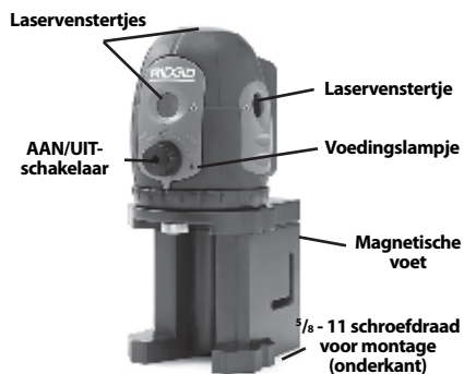
Figuur 2 – Laseronderdelen
