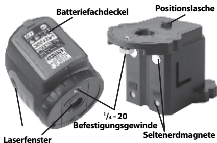
Abbildung 3 - Laserteile
