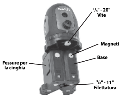
Figura 6 - Base
