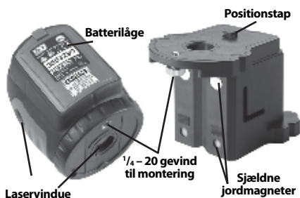
Figur 3 - lasernivelleringsdele
