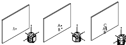
Rysunek 9 - Automagiczne sprawdzenie 3 promieni poziomych
