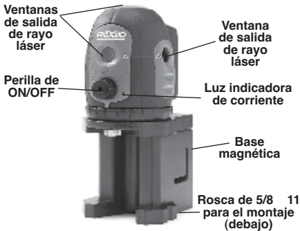
Figura 2 Piezas del Láser
