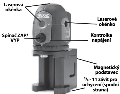
Obrázek 2 – Součásti laseru
