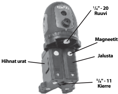
Kuva 6 - Jalusta
