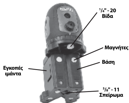
Εικόνα 6 - Βάση
