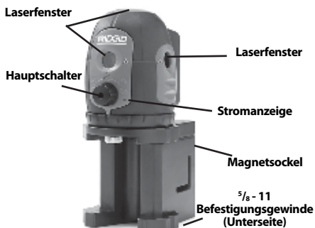
Abbildung 2 - Laserteile
