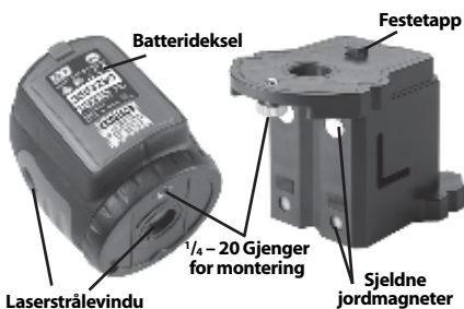
Fig. 3 - Laserdeler, nivellering
