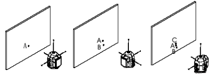
Şekil 9 - 3 Yatay Işının Kendini Kontrol Etmesi
