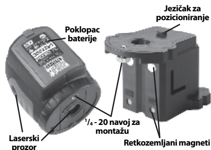
Slika 3 - Delovi za nivelisanje lasera
