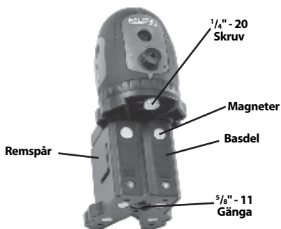
Figur 6 - Bas
