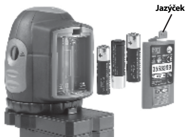
Obrázek 4 - Instalace baterií
