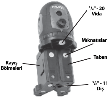
Şekil 6-Taban
