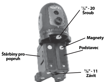
Obrázek 6 - Podstavec
