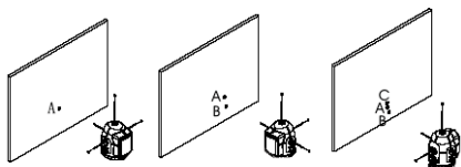
Рис. 9 - Самопроверка 3-х горизонтальных лучей лазера
