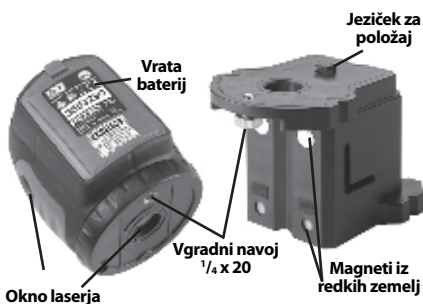
Slika 3 – Deli laserja
