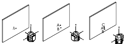
Obr. 9 - Kontrola troch horizontálnych lúčov
