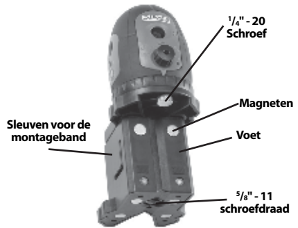
Figuur 6 – Voet
