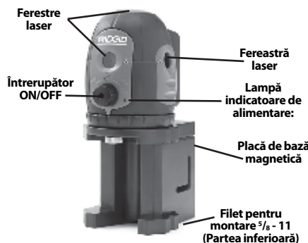
Figura 2 - piese laser
