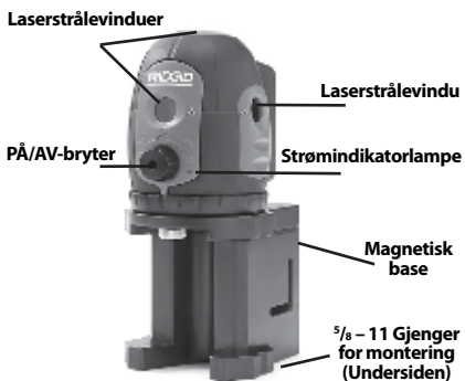
Fig. 2 - Laserdeler
