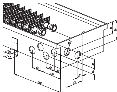
KORAFLEX FI 13/34
