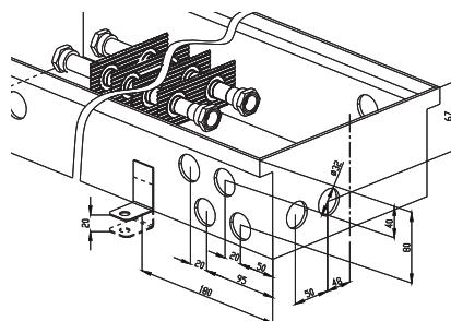
KORAFLEX FW 13/34
