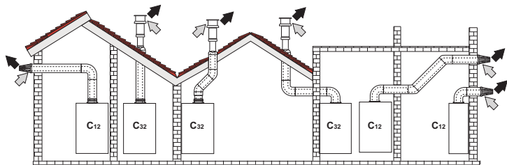
мал. 21 - Приклад підключення за допомогою співісних (коаксимальних) труб (⇐ = Повітря / ⇨ = Відпрацьовані гази)
