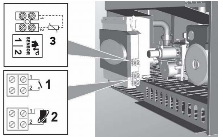
fig. 20 - Acceso a la regleta de conexiones
