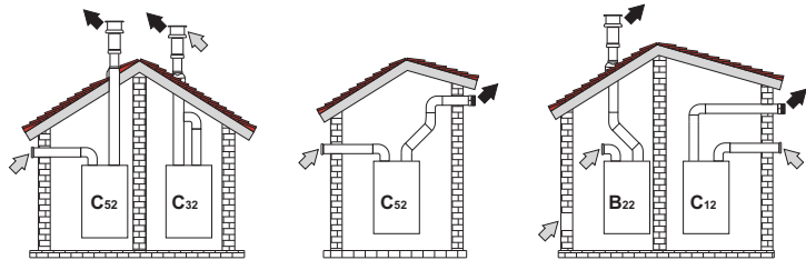
мал. 23 - Приклад підключення за допомогою відокремлених труб (⇐ = Повітря / ⇨ = Відпрацьовані гази)
