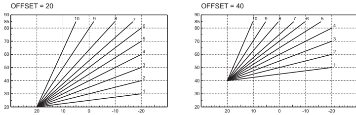
мал. 15 - Пиклад паралельного пересування компенсаційних кривих
