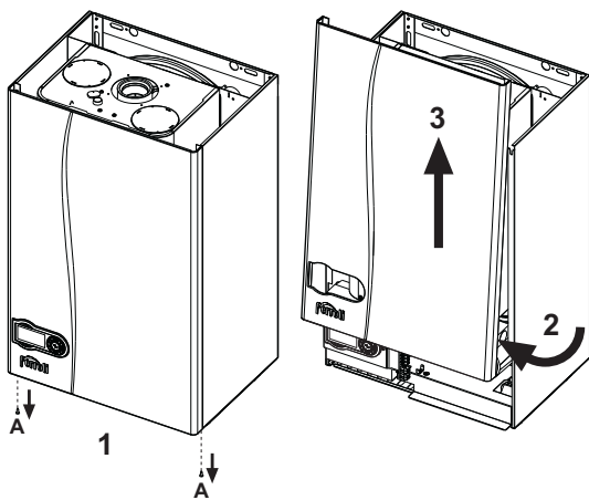
fig. 28 - Deschiderea carcasei
