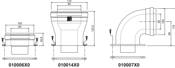
şek. 22 - Koaksiyal kanallar için çıkış aksesuarları
