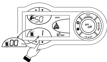
fig. 26 - Modalidad TEST (potencia de la calefacción = 100%)
