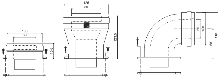
fig. 22 - Accessoires de départ pour conduits coaxiaux
