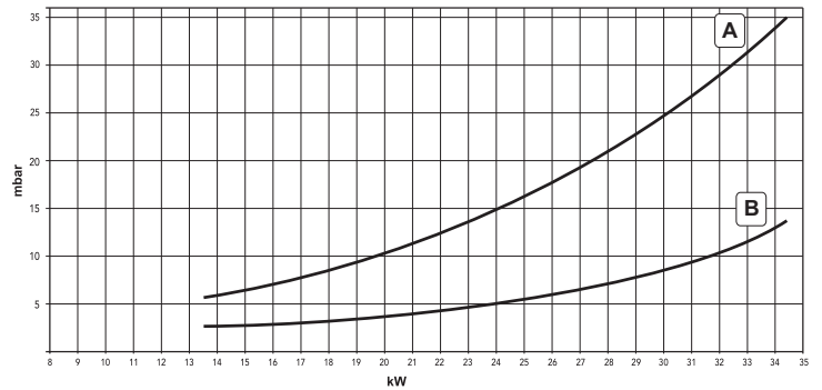
fig. 35 - Diagramma pressione/potenza DIVAtop MICRO F 32
