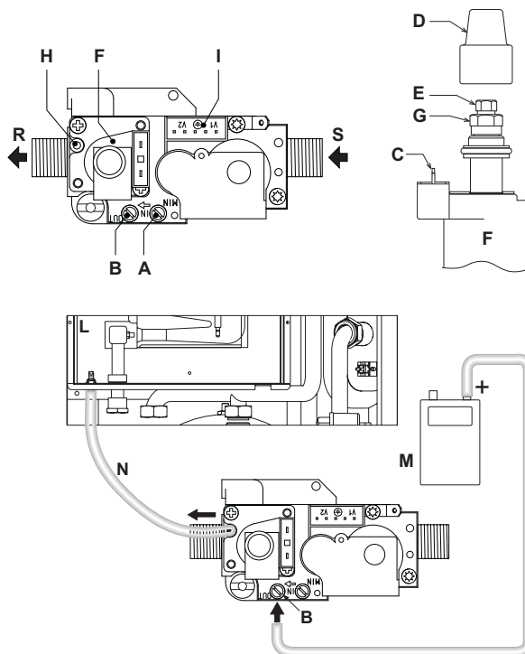
рис. 27 - Газовый клапан
