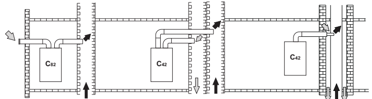
fig. 25 - Exemples de raccords à l'aide de tuyaux coaxiaux (⇨ = Air / ⇨ = Fumées)
