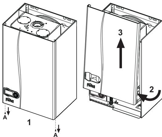
fig. 28 - Démontage de l'habillage
