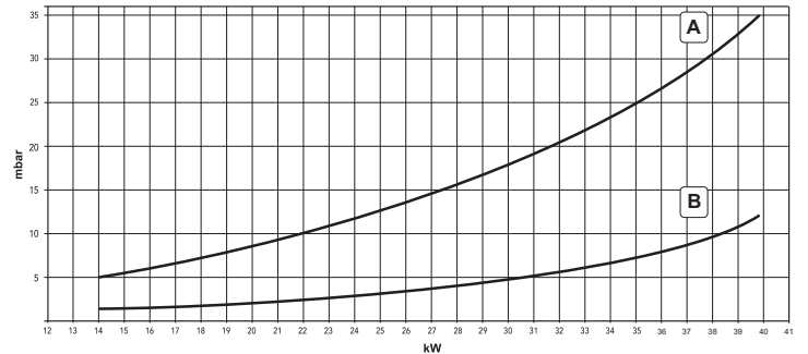
fig. 37 - Diagramma pressione/potenza DIVAtop MICRO F 37
