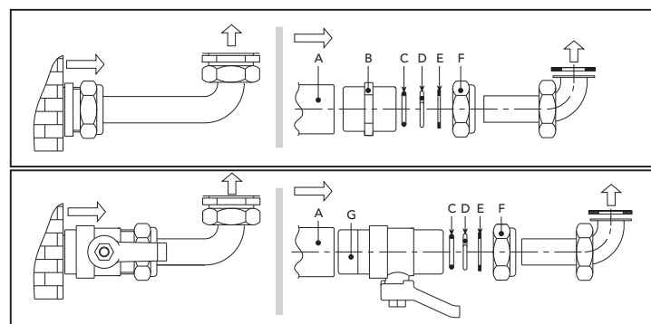
fig. 18 - Kit de racordare
