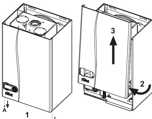
рис. 28 - Снятие кожуха
