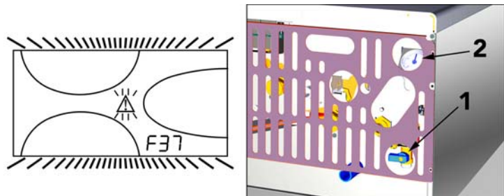
fig. 16 - Anomalia pressione impianto insufficiente
