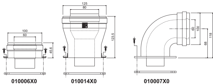
мал. 22 - Початкові елементи для коаксимальних трубопроводів
