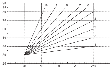
fig. 14 - Curbe de compensare
