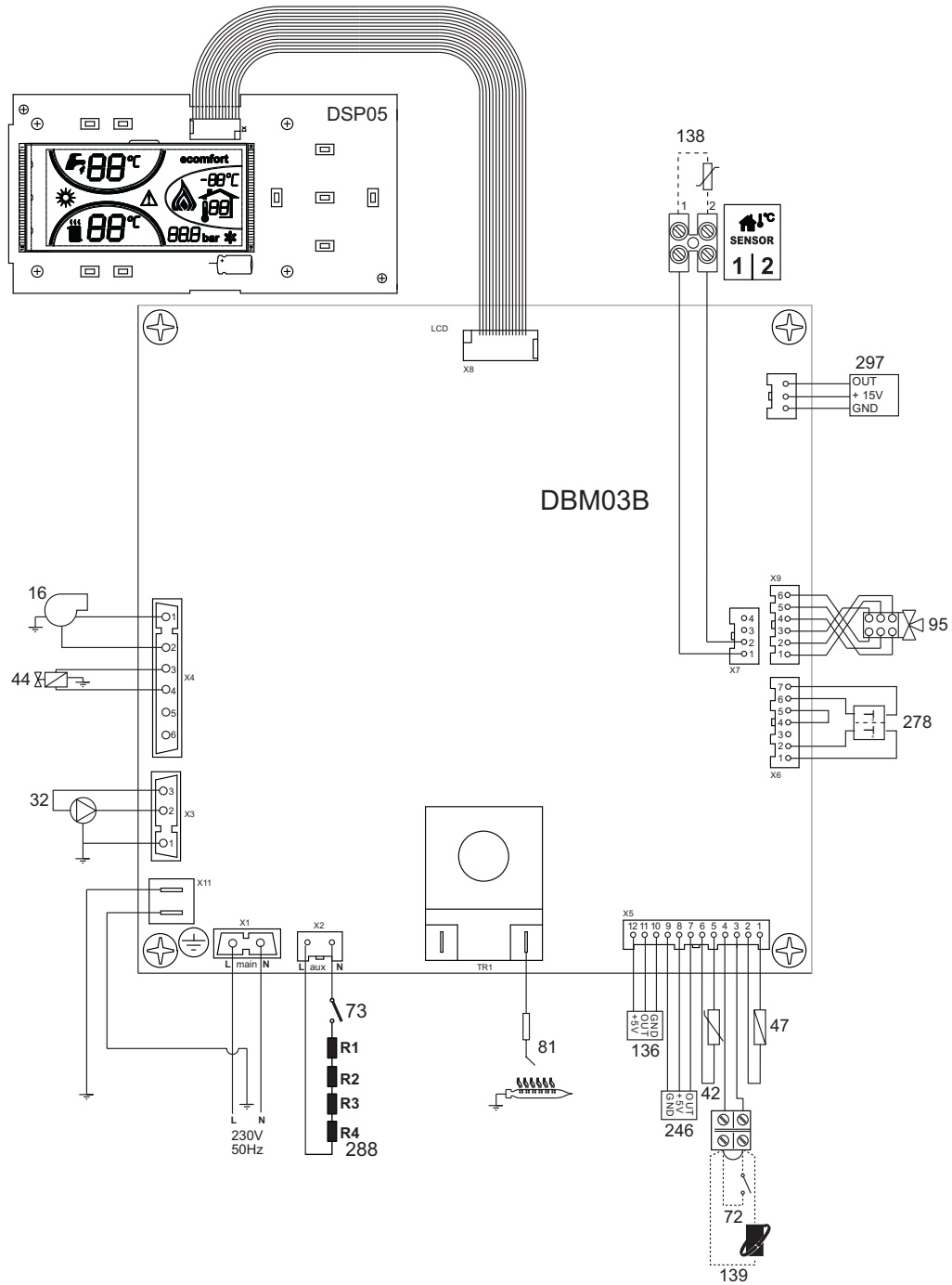
fig. 39 - Schemă electrică
