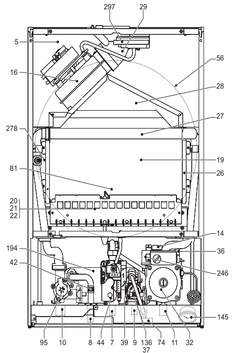
мал. 32 - Загальний вигляд DIVAtop MICRO F 37
