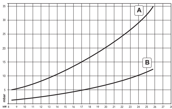
fig. 33 - Diagramă presiune/putere DIVAtop MICRO F 24
