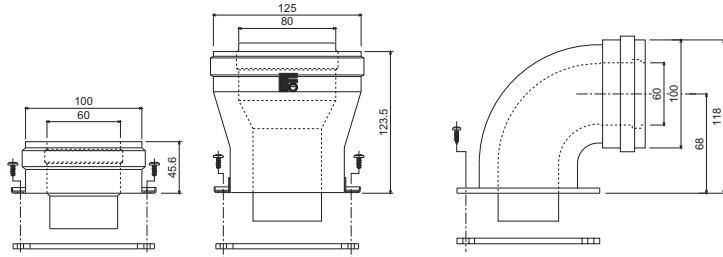
рис. 22 - Исходные элементы для коаксиальных воздухопроводов
