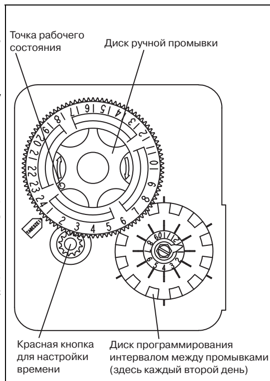
Рис. 10: Таймер (спереди)
