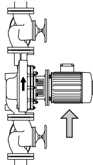
Рисунок 5: Обеспечить опирание двигателя
