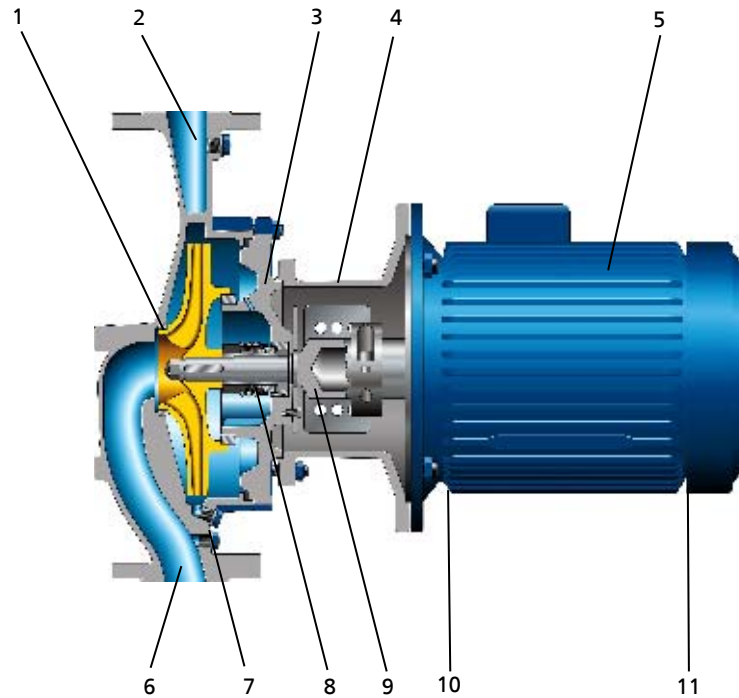
Рисунок 4: Сечение
