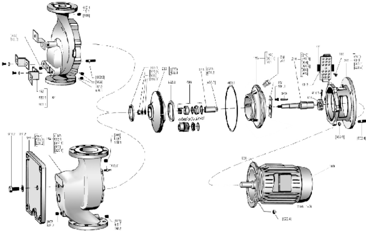
Рисунок 13: Стандартное торцевое уплотнение и зажимная напорная крышка
