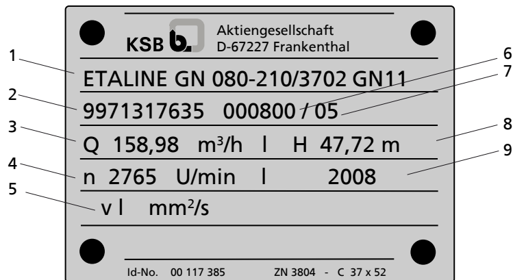
Рисунок 3: Заводская табличка
