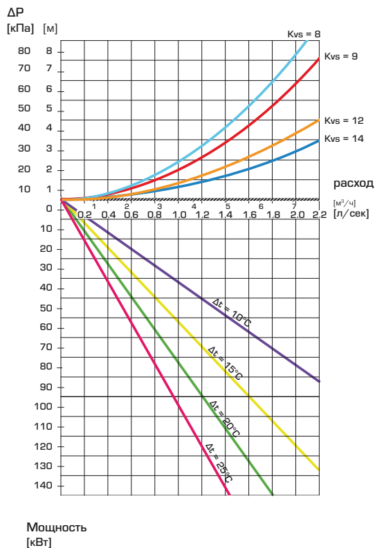
VTC500 – потеря давления
