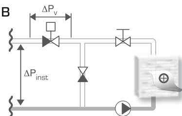
Установка с местным циркуляционным насосом
