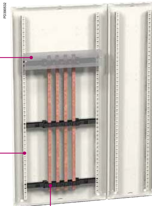
Изолирующий экран для защиты от прямого прикосновения к соединениям
