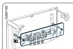
Изолирующий экран для защиты от прямого прикосновения к соединениям
