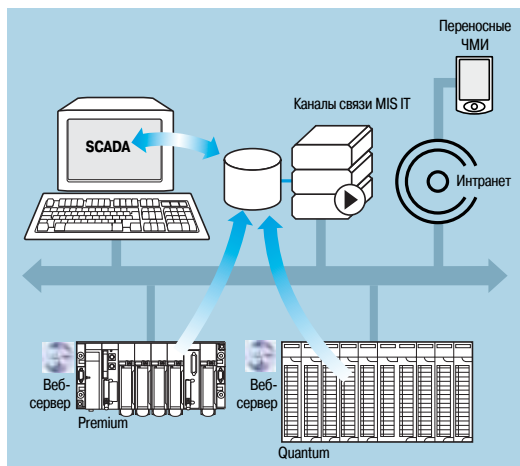
Смешанные архитектуры
