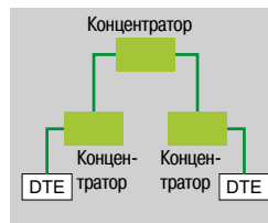
Топология «дерево»
