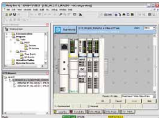
Редактор DTM (площадка Modicon STB)
