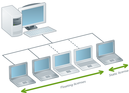
Архитектура для одного сервера с 2 плавающими лицензиями Control Client и 1 статической лицензией
