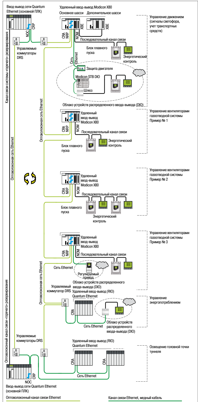
Архитектура ввода-вывода Quantum Ethernet с «горячим» резервированием: управление автодорожным туннелем
