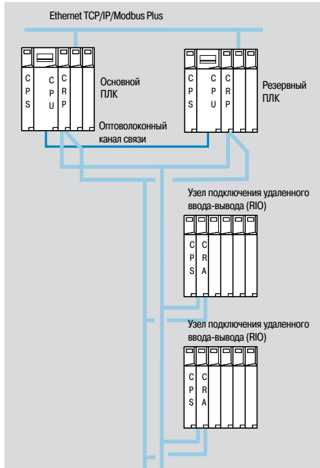
Система «горячего» резервирования и узлы RIO
