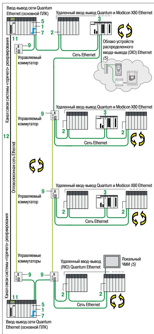
Архитектура ввода-вывода с «горячим» резервированием Quantum Ethernet для больших расстояний
