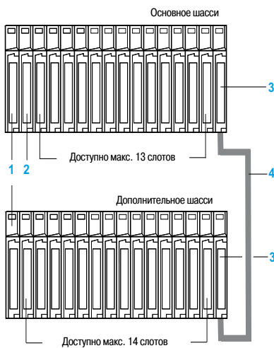
Архитектура локального ввода-вывода
