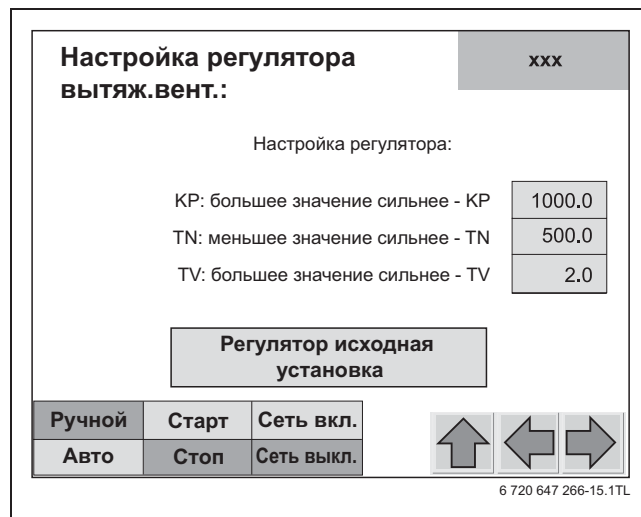
Рис. 34 Экран "Настройка регулятора вытяжного вентилятора"
