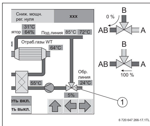
Рис. 36 Проход воды через трёхходовой клапан
