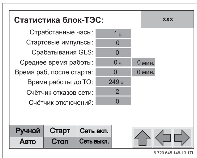
Рис. 45 "Статистика блок-ТЭС"
