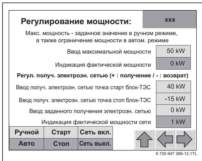
Рис. 30 Экран настройки "Регулирование мощности"
