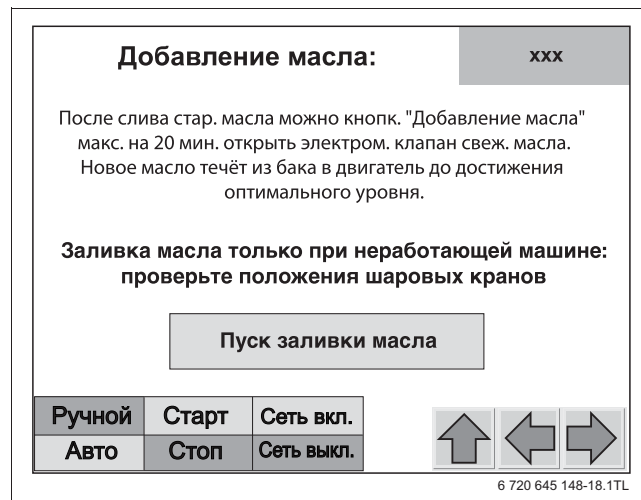
Рис. 42 Экран настройки "Добавление масла"
