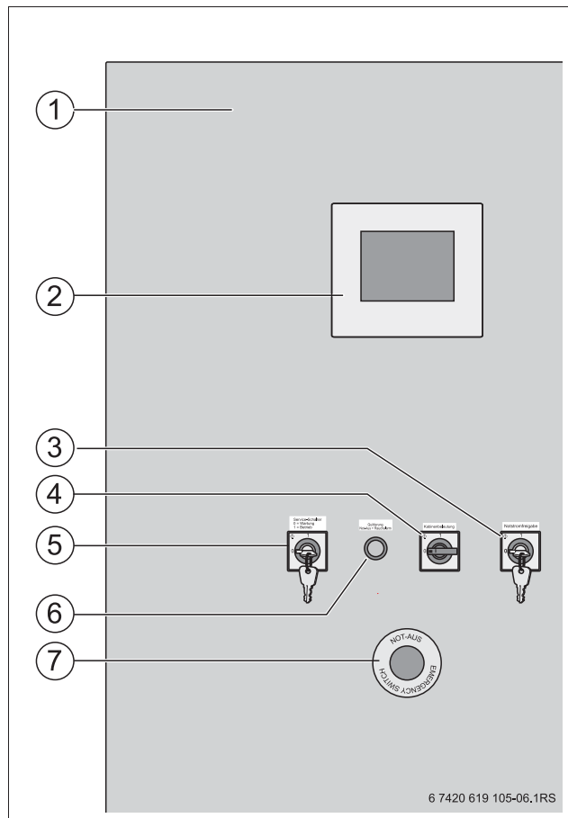
Рис. 4 Часть электрошкафа с элементами управления
