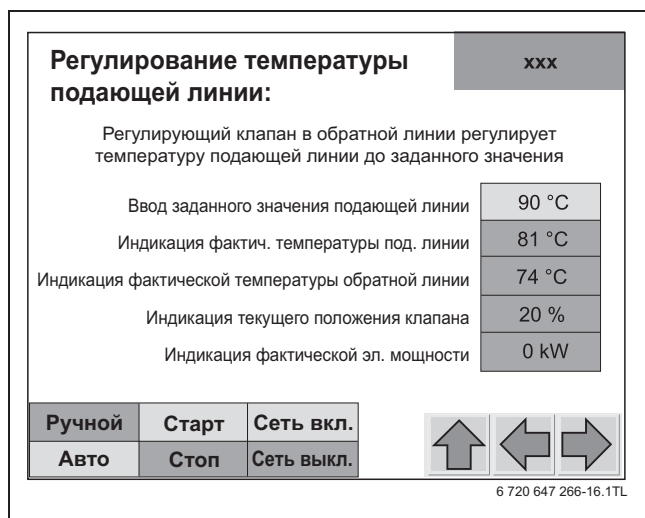
Рис. 35 Экран настройки "Регулирование температуры подающей линии"
