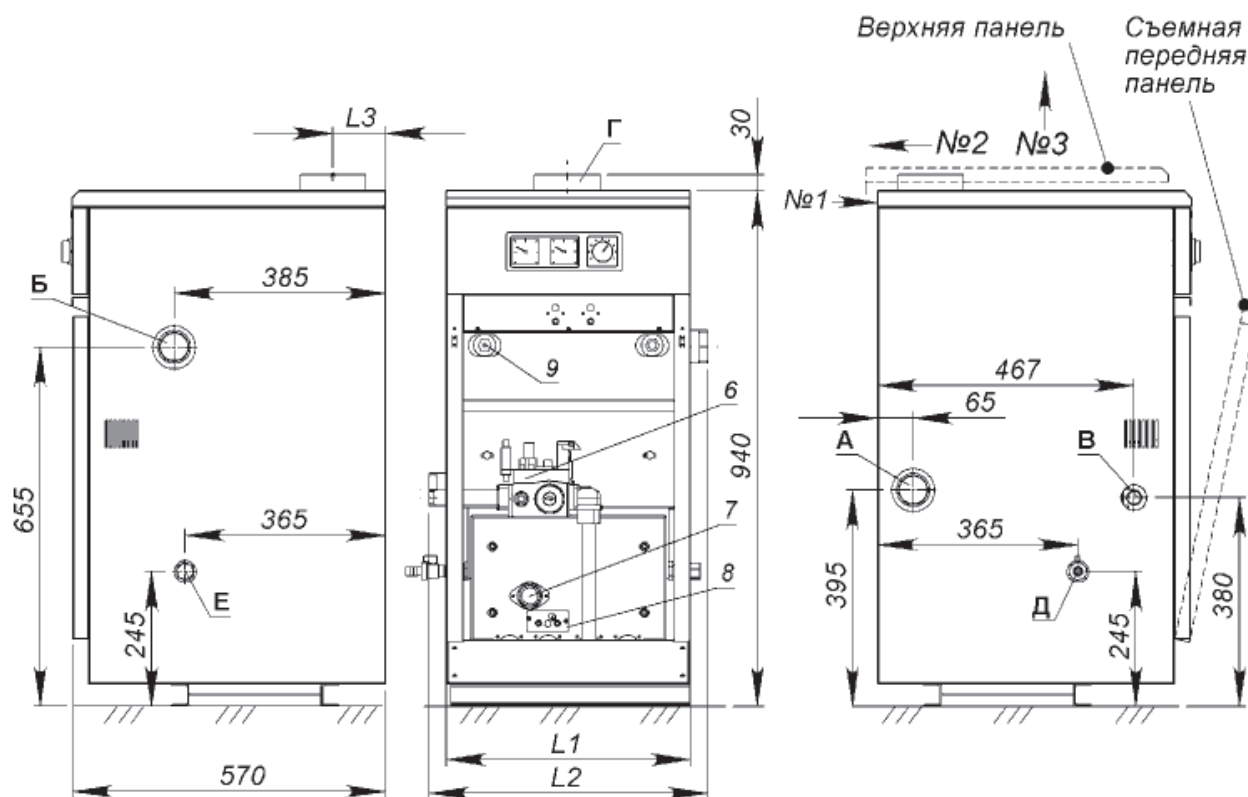
Рисунок 2. Внешний вид, габаритные и присоединительные размеры котла ALFA COMFORT v15.
