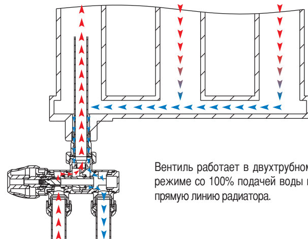
Двухтрубный режим
