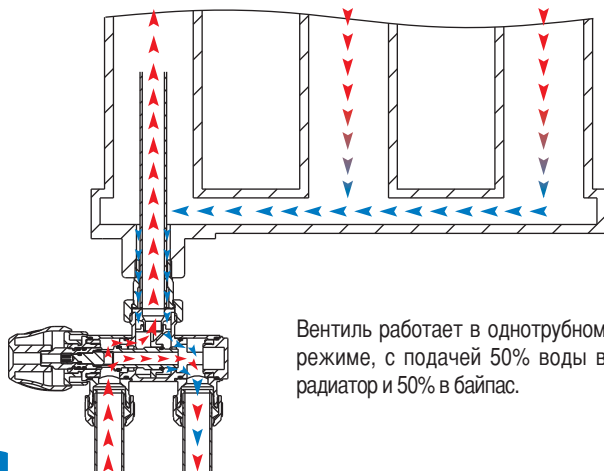
Однотрубный режим
