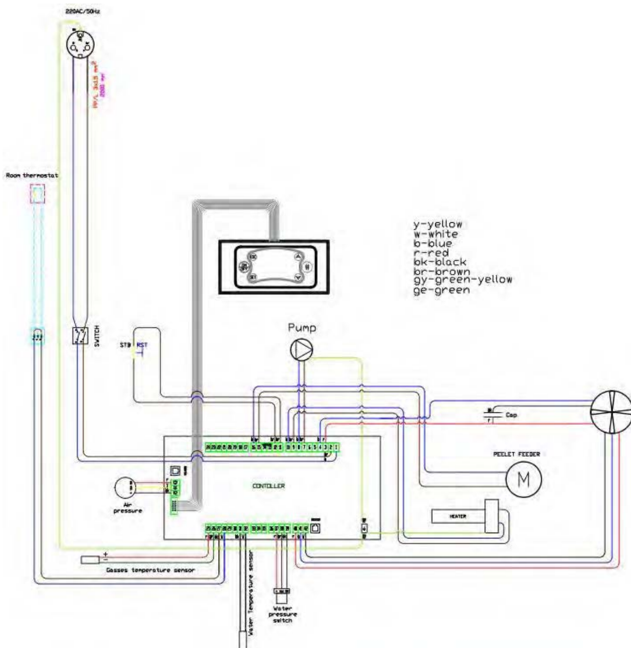
Рис 10. Электрические подключения
