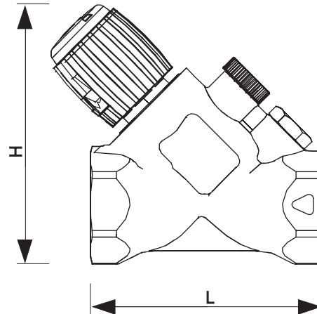
Рис. 2 Вид сбоку
