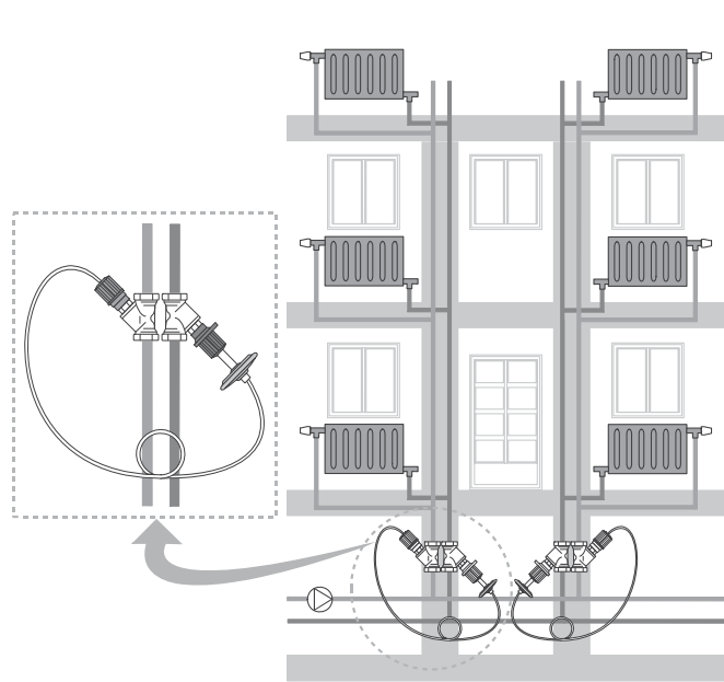
Рис. 2. Stop Valve-3 в качестве запорного клапана подающей магистрали с подключенной импульсной трубкой от мембранного модуля Kombi-DU, установленного на клапан Kombi-3-plus СИНИЙ в двухтрубной системе
