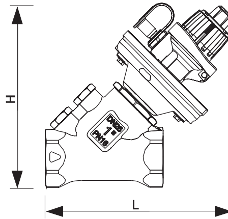
Рис. 2 Вид сбоку
