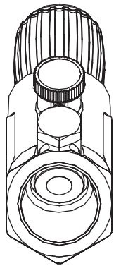
Рис. 1 Вид спереди
