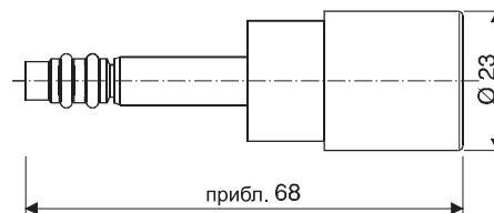
Рис. 4. Термальный привод для Alwa Kombi-4
