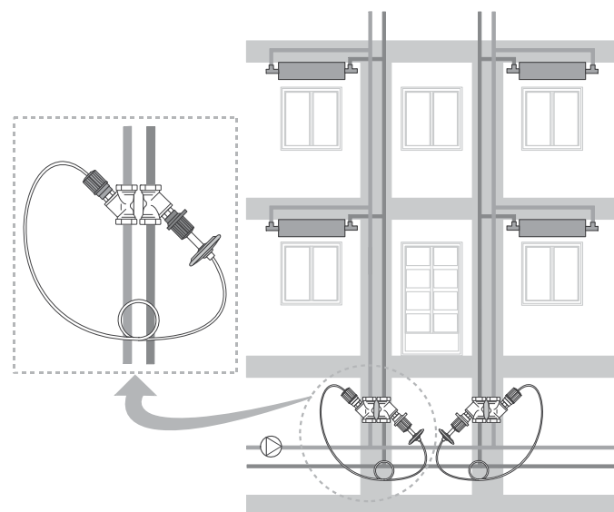
Рис. 3. V5012C Kombi-DU в системе охлаждения
