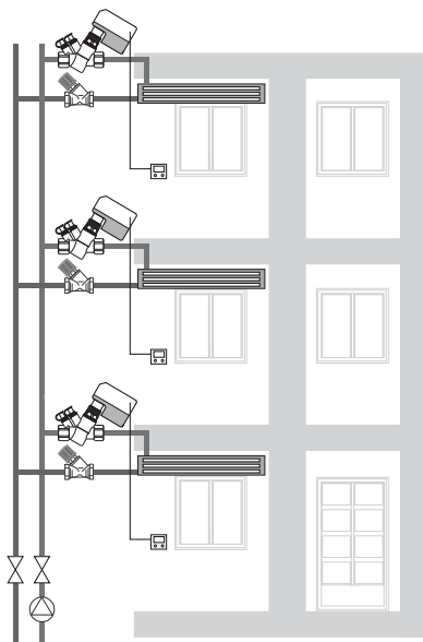
Рис. 3 Фен-койл, 2-трубная система
