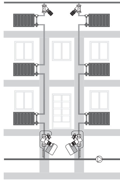
Рис. 5 Отопление, 1-трубная вертикальная система
