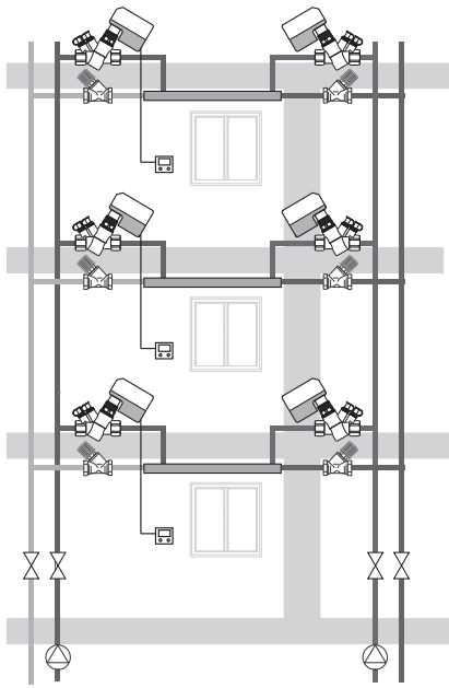
Рис. 4 Потолочное охлаждение, 4-трубная система
