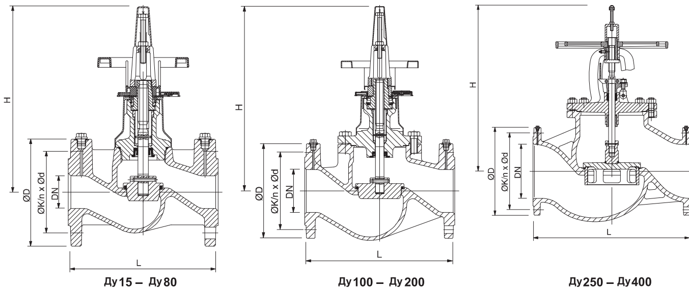
Рис. 1. Размеры клапанов Kombi-F-II
