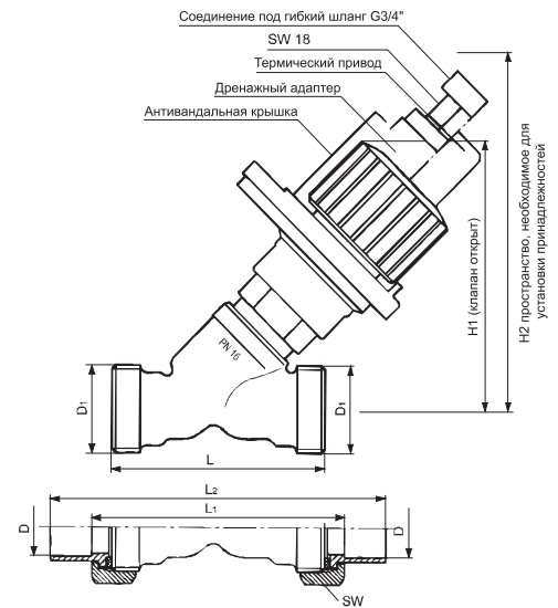
Рис. 3. Alwa-Kombi-4 с наружной резьбой
