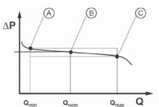
Рис. 6 Регулировочная характеристика
