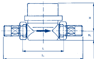
Счетчик воды E-T Domagua m
