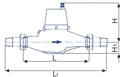
Рис.1 Крыльчатый расходомер М-Т с резьбовым соединением для горизонтального монтажа
