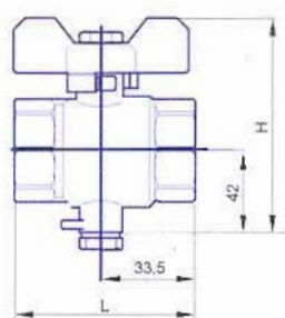
Шаровой кран со встроенным термодатчиком
