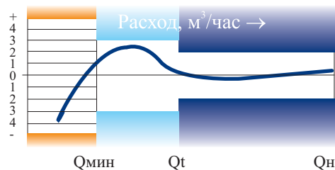
Кривая погрешности измерений
