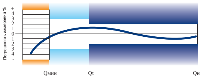
Типичная кривая погрешности измерений
