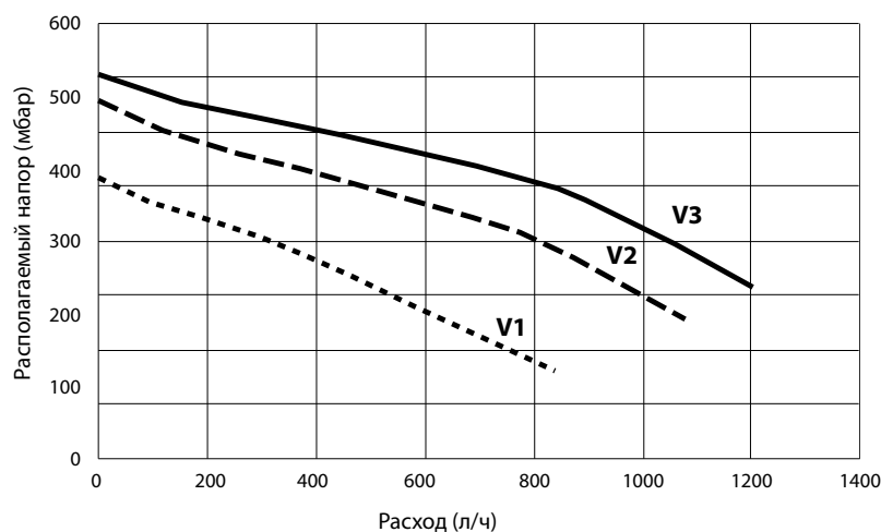
НАСОС НИЗКОТЕМПЕРАТУРНОГО КОНТУРА ЗОНЫ 2
