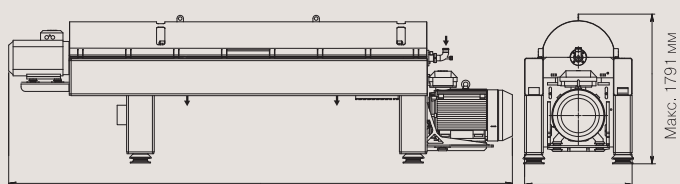
ALDEC G2-95 5462 mm 1150 mm ALDEC G2-115 6402 mm 1450 mm
