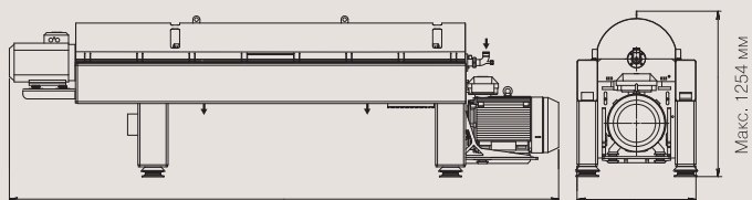
ALDEC G2-45 4273 mm 990 mm
