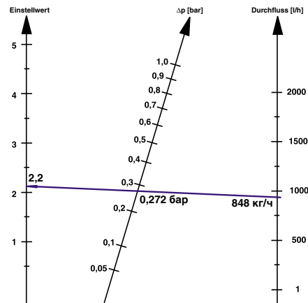
Рис.4.89. Определение значения гидравлической настройки ( n=2,2 ) перепускного клапана ГЕРЦ 4004, d20, арт.1400442 (поз.16 рис.4.74 ветки «В») при задаваемых расчетных значениях G_{\text{нomp}}=848 \text{ кг/ч} и \Delta P_{\text{заг}}=0,272 \text{ бар} .
