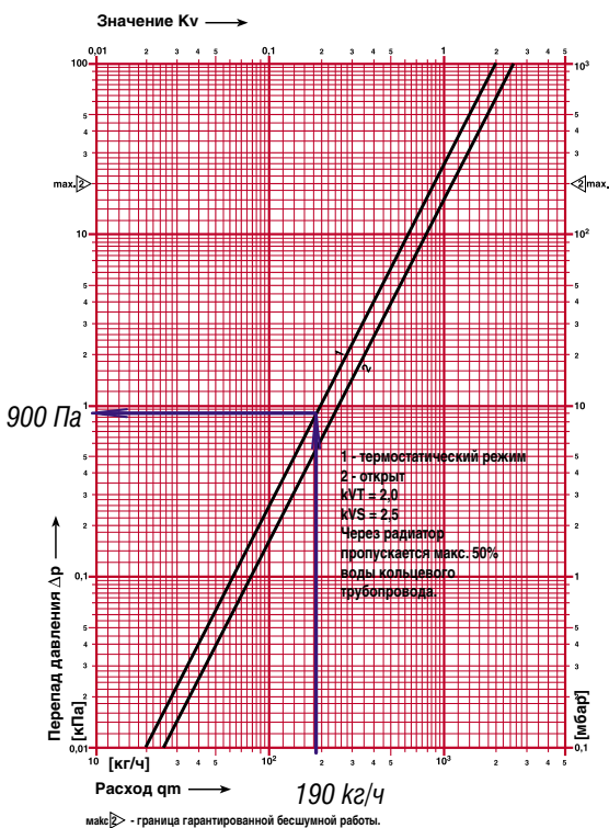
Рис. 4.99. Определение \Delta P_{\text{кл1}} узла подключения ГЕРЦ-2000 (поз.2.5 рис.4.97)
