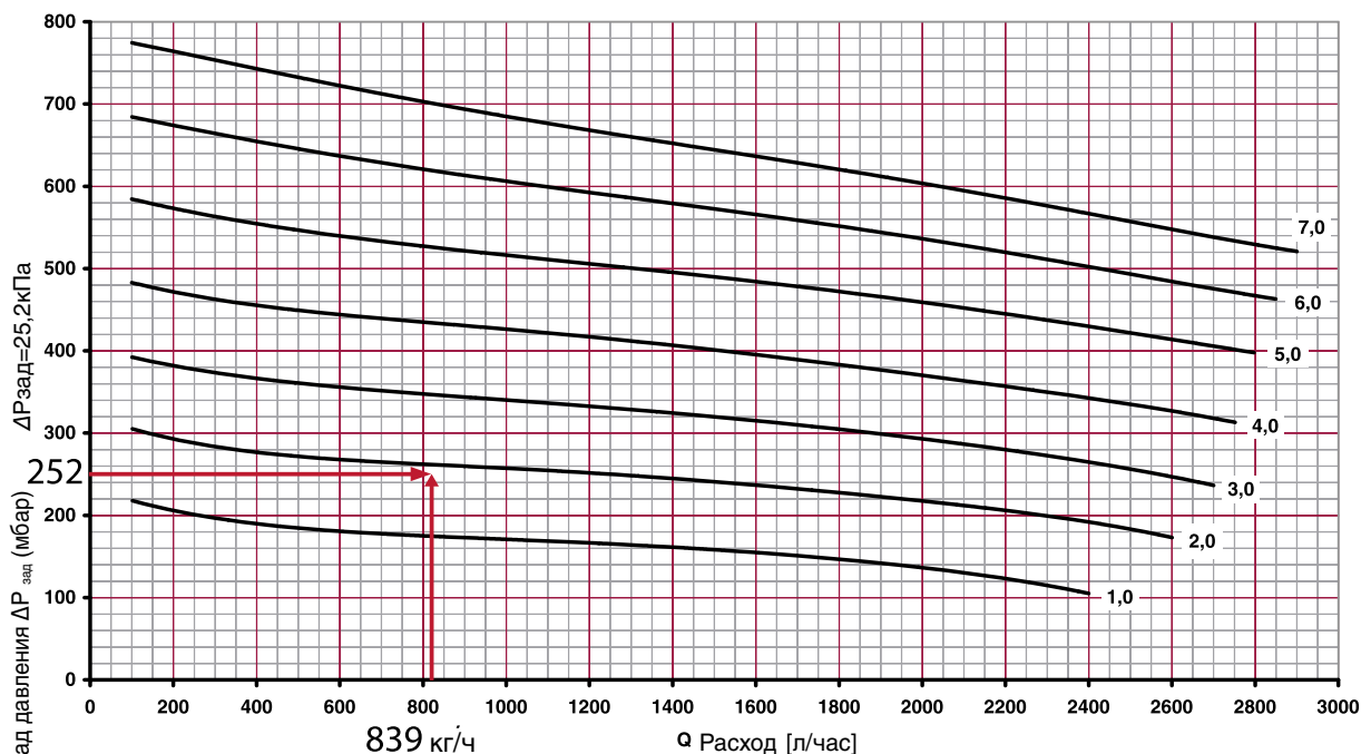
Рис. 4.73. Определение значения гидравлической настройки (n=1,9) регулятора перепада давления ГЕРЦ 4002, d25, арт.1400243 (поз.8 рис.4.59 ветки «В») при задаваемых расчетных значениях G_{потр}=839\text{кг/ч} и \Delta P_{зад}=25,2\text{кПа}
