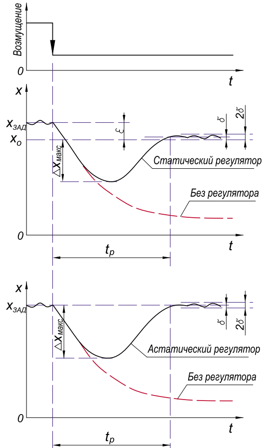
Рис.2.2. График переходного процесса регулирования при скачкообразном уменьшении возмущающего воздействия с показателями качества регулирования
