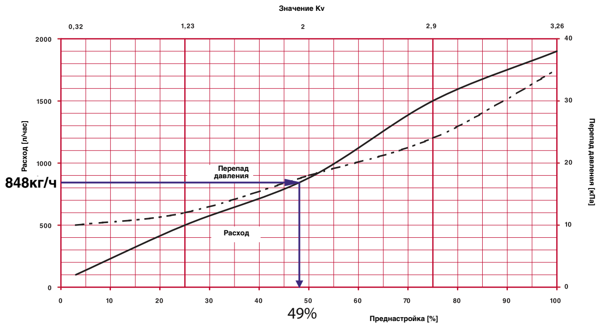
Рис. 4.90. Определение значения гидравлической настройки регулятора расхода ГЕРЦ 4001, d25, арт.1400123 (поз.8 ветки «В» рис.4.74 при расчетном значении G_{общ} = 848 \text{ кг/ч} ).
