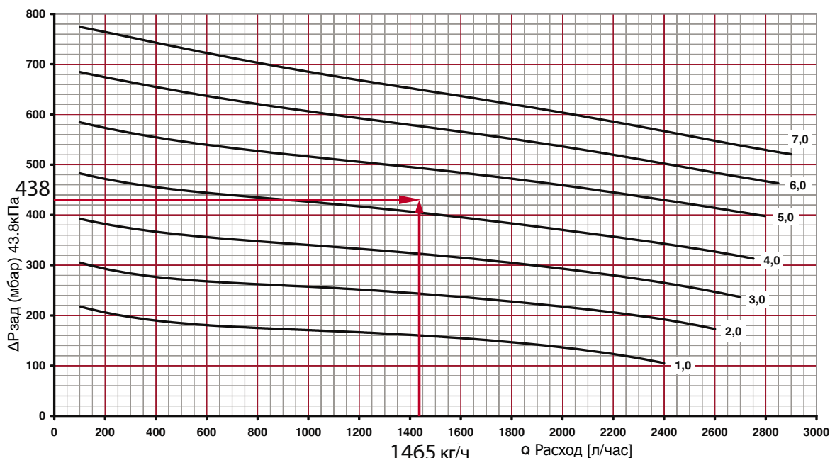
Рис.4.81. Определение значения гидравлической настройки ( n=4,6 ) регулятора перепада давления ГЕРЦ 4002, d25, арт.1400263 (поз.15 рис.4.74 ветки «А») при задаваемых расчетных значениях G_{потр}=1465\text{кг/ч} и \Delta P_{зад}=43.8\text{кПа}
