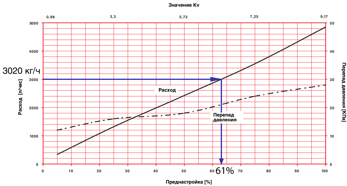
Рис. 4.25. Определение значения гидравлической настройки регулятора расхода ГЕРЦ 4001, d50, арт.1400126 (поз.3 рис. 4.23 для воздухоохладителя установки П2 при расчетном значении G_{общ} = 3020 \text{ кг/ч} .)
