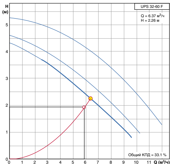
Рис. 4.18. Расчетная характеристика смесительного насоса UPS 32-60F (поз. 7 рис. 4.15)
