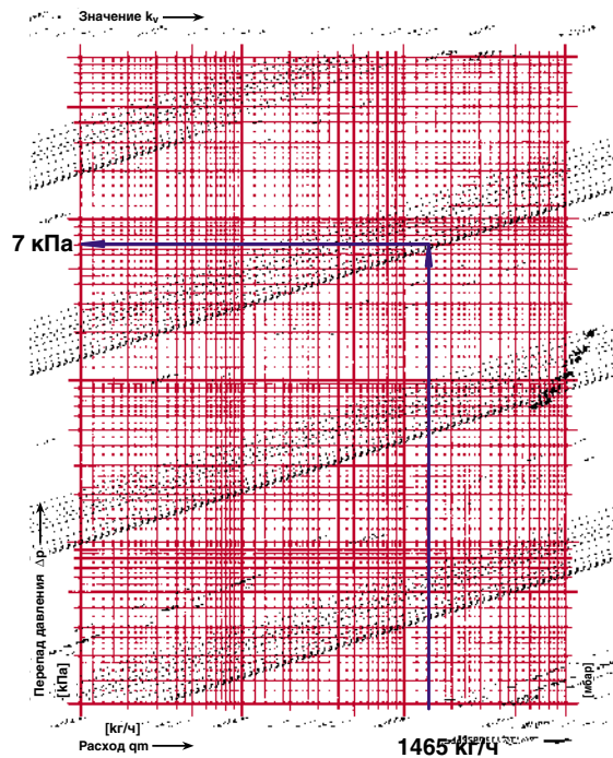
Рис. 4.75. Определение сопротивления вентиля балансового ШТРЕМАКС-GM, d32, арт.1421704 с измерительными клапанами, поз.7 рис. 4.74.
