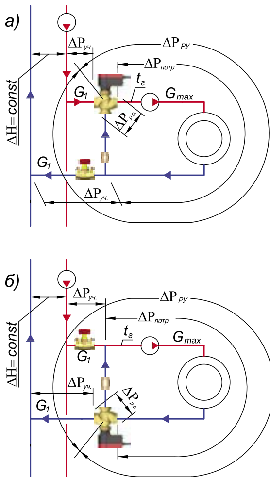
Рис. 3.15. Расчетная первая схема узла смешения со смесительным насосом на магистральном теплопроводе системы теплотребления
