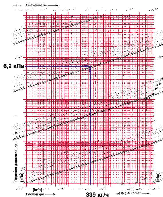
Рис. 4.71. Определение гидравлической преднастройки балансового вентиля ШТРЕМАКС-GM, d20, арт.1421702 поз.12 фэнкойла №10 для создания сопротивления 6,2кПа при расходе теплоносителя 339кг/ч.
