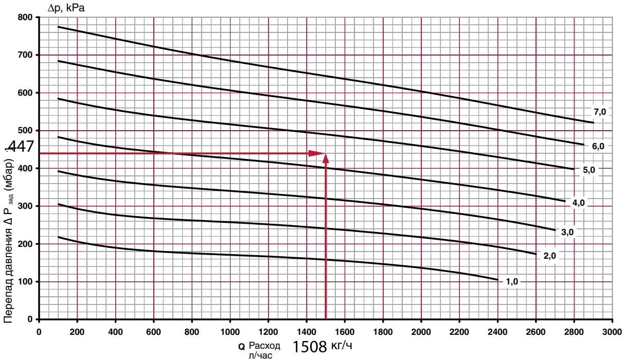
Рис. 4.66. Определение значения гидравлической настройки ( n=4.7 ) регулятора перепада давления ГЕРЦ 4002, d25, арт.1400263 (поз.8 рис.4.59 ветки «А») при задаваемых расчетных значениях G_{\text{номр}}=1508 \text{ кг/ч} и \Delta P_{\text{заг}}=44.7 \text{ кПа}
