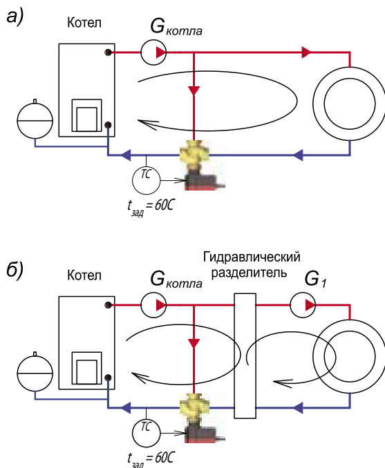
Рис. 4.41. Общая схема системы теплотребления
