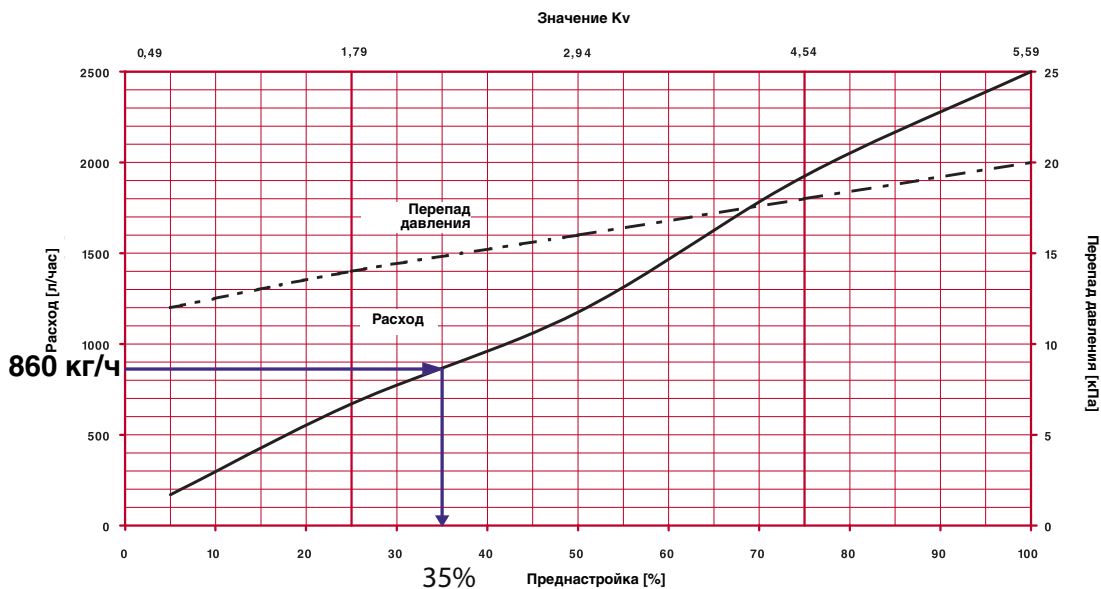
Рис.4.96. Определение значения гидравлической настройки регулятора расхода ГЕРЦ 4001, D32, арт.1400123 (поз.8 рис.4.91 на системе отопления аудитории №5) при расчетном значении G_{общ} = 860 \text{ кг/ч} .
