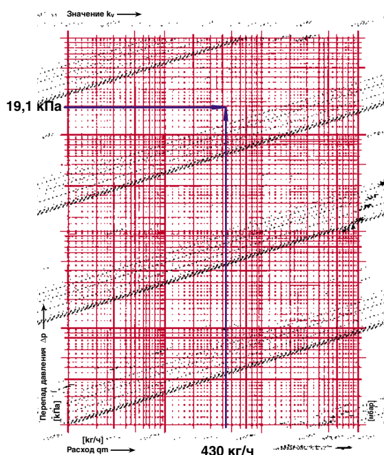
Рис. 4.80. Определение гидравлической преднастройки балансового вентиля ШТРЕМАКС-GM, d20, арт.1421702 поз.12 фэнкойла №1 для создания сопротивления 19,1кПа при расходе воды 430кг/ч.
