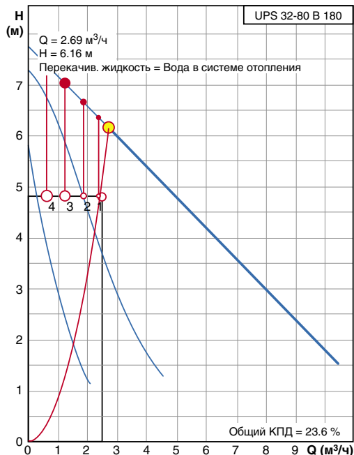
Рис. 4.38. Расчетная характеристика смесительного насоса UPS 32-80 В 180 (поз.Р3.1 рис.4.28)
