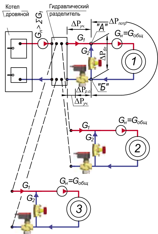
Рис.3.13. Расчетная вторая схема для узлов смешения со смесительным насосом на магистральном теплопроводе системы теплоснабжения (при параллельном присоединении систем теплоснабжения к гидравлическому разделителю)
