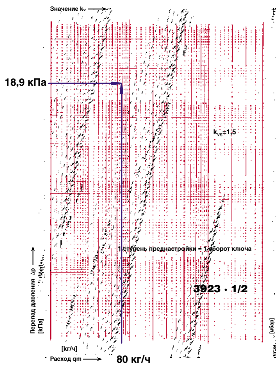
Рис.4.102. Определение значения гидравлической преднастройки вентиля балансового ГЕРЦ RL-5, арт.1392301, d15 (поз.3.1 рис.4.97) при значениях P_{6.8.3.1}=18,9\text{кПа} и G_{6.8.3.1}=80\text{кг/ч} .
