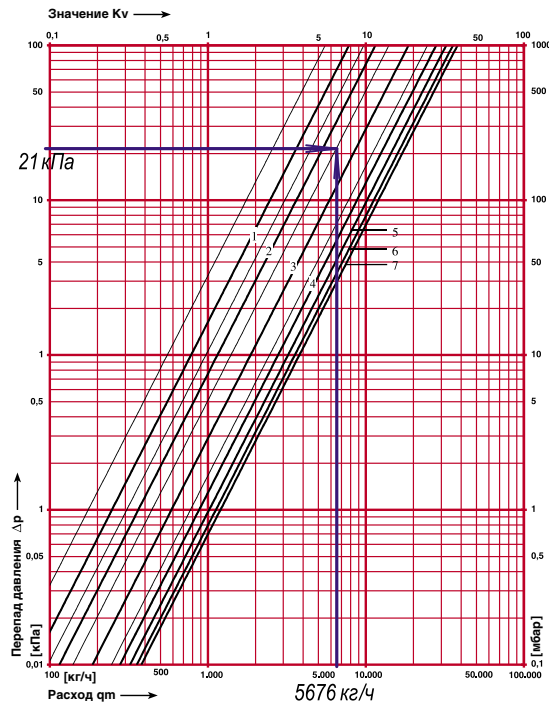
Рис.4.95. Определение значения гидравлической преднастройки вентиля балансового фланцевого ШТРЕМАКС-GMF, d50 с измерительными клапанами, арт.1421846 (поз.4 на теплопроводе T2* рис.4.91) при расчетных значениях \Delta P_{\beta,4^*}=21,0\text{кПа} и G_{\beta,4^*}=5676\text{кг/ч} .
