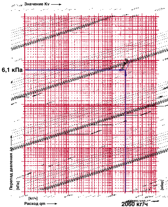
Рис. 4.51. Определение значения гидравлической преднастройки вентиля балансового ШТРЕМАКС-GM, d25, арт.1421703 с измерительными клапанами, поз.2.1 рис.4.46.
