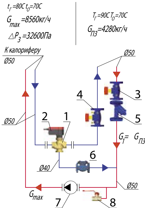
Рис. 4.19. Узел регулирования «3»
