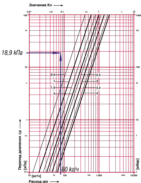
Рис.4.101. Определение значения гидравлической преднастройки вентиля балансового ШТРЕМАКС 4017М арт.1401711, d15 с измерительными клапанами, (поз.3.1 рис.4.97) при значениях \Delta P_{6.8.3.1}=18,9\text{кПа} и G_{6.8.3.1}=80\text{кг/ч} .
