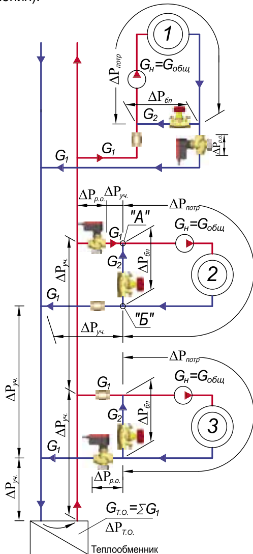
Рис. 3.12. Расчетная вторая схема для узлов смешения со смесительным насосом на магистральном трубопроводе системы теплоснабжения (при параллельном присоединении систем теплоснабжения к теплообменнику или к газовому котлу)
