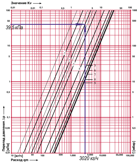
Рис 4.24. Определение значения гидравлической преднастройки вентиля балансового фланцевого ШТРЕМАКС-GMF, d40 с измерительными клапанами, арт.1421845 (поз.5 рис.4.23) при расчетных значениях \Delta P_{в.5} = 39,5 \text{ кПа} и G_{в.5} = 3020 \text{ кг/ч} .
