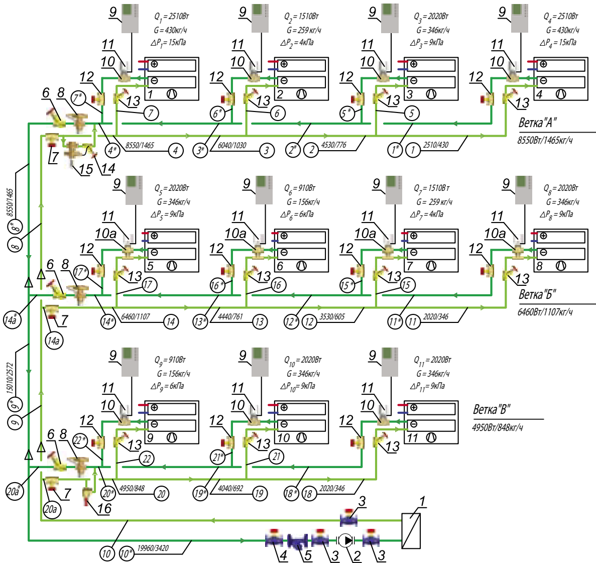
Рис. 4.74. Схема расчетная системы холодоснабжения четырехтрубных фэнкойлов
