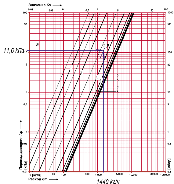
Рис. 4.5. Определение гидравлических характеристик вентиля балансирового фланцевого ШТРЕМАКС-GMF, d25 с измерительными клапанами, арт.1421843 (поз.13а рис.4.1).
