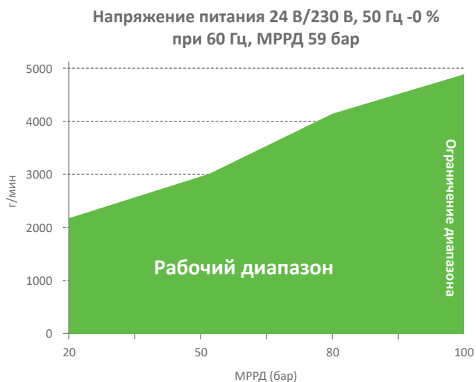
Рис. 1: OM5: Эксплуатационные показатели в зависимости от напряжения питания: Разница в скорости потока и давлении между входом и выходом (тип масла Reniso C85E, температура масла 54 °C)
