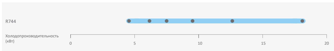
Компрессор Copeland Stream для низкотемпературных применений на R744: надежность и лучшая в своем классе производительность для субкритических циклов
