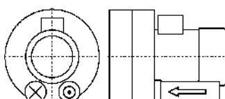
Fig. 2: Turbinas de canal lateral de doble etapa (2 rodetes en paralelo) Double stage side channel blower (2 impellers in parallel) Series: HPExxxx-2P... Двухступенчатые турбокомпрессоры (2 рабочих колеса, патрубки расположены параллельно) Серии: HPExxxx-2P...
