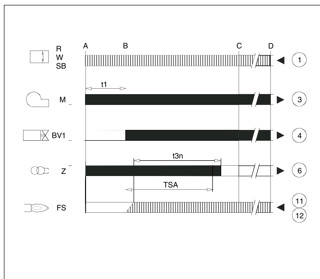
Рис. 9 Выполнение программы автомата горения дизельного топлива
