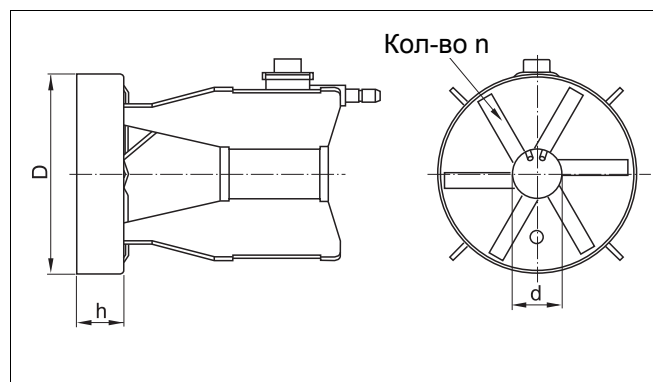
Рис. 2 Распределительный диск
