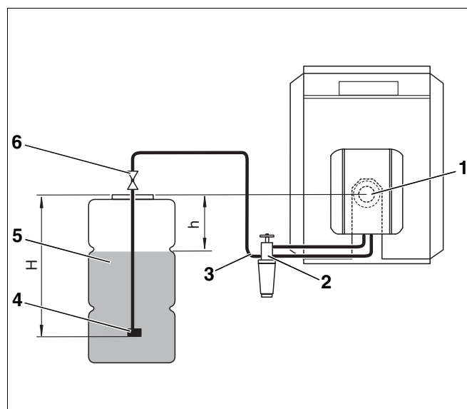
Рис. 38 Топливный бак установлен ниже топливного насоса
