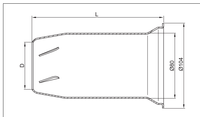
Рис. 3 Труба горелки
