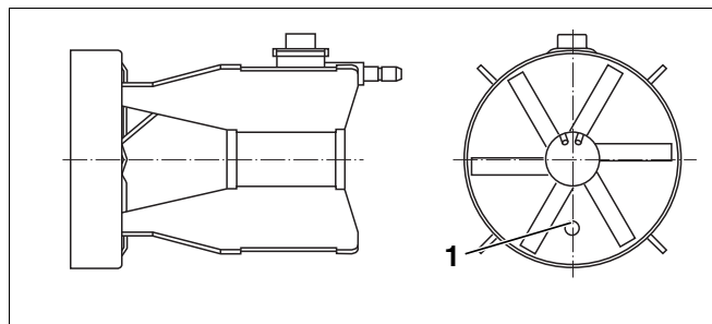
Рис. 31 Распределительный диск
