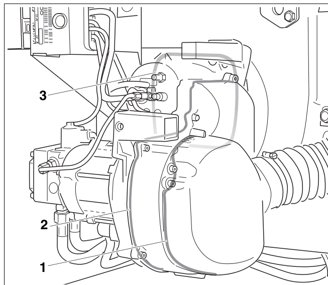
Рис. 33 Дополнительное уплотнение Logatop SE RLU
