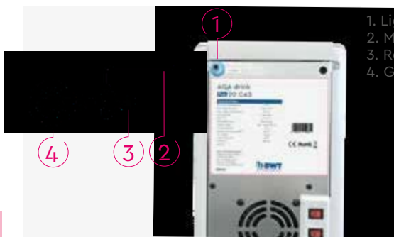
Fig. 8: Ligar a garrafa de gás comprimido de CO 2
