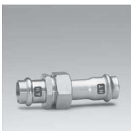
Номер по каталогу и название 18330 – сгон ВПр-ВПр с плоским уплотнением
