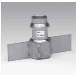
Номер по каталогу и название 17270F – муфта переходная ВПр-ВР с креплением
