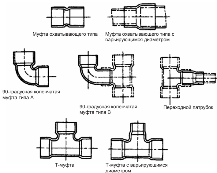
Рис. 2: муфтовые соединения
