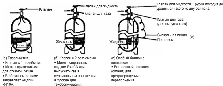
Рис. 8: типы баллонов
