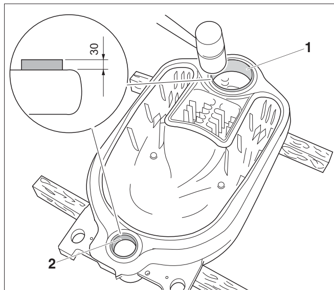
Рис. 8 Установка ниппеля
