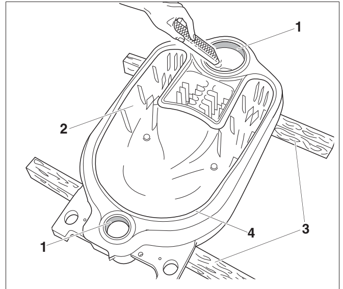
Рис. 6 Удаление заусенцев
