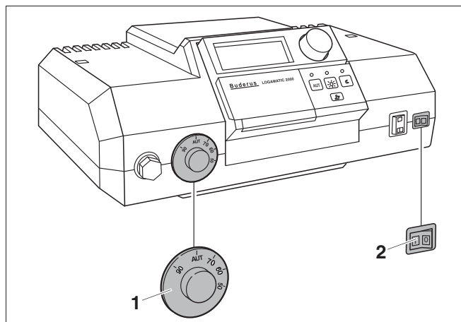
Рис. 67 Включение системы управления (например, Logomatic 2000)
