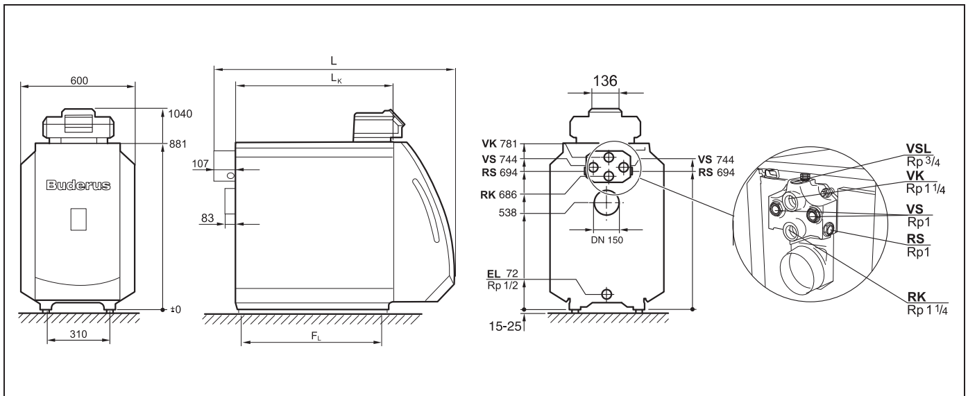
Рис. 2 Подключения и размеры (приведены в мм)
