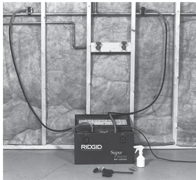
Figuur 6 – Toepassing met twee vriescoppen
