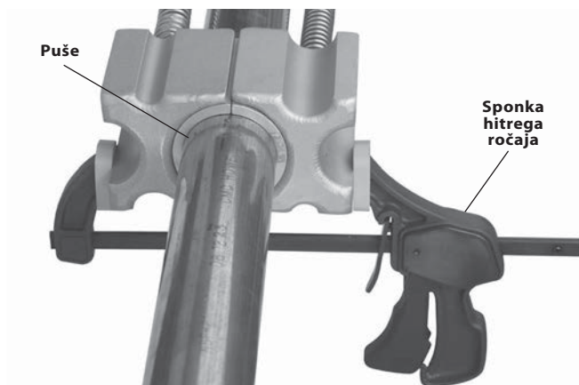
Slika 4 – Namestitev zamrzovalne glave s sponko hitrega ročaja
