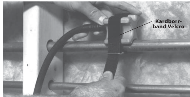
Figur 5 – Fästa fryshuvudet med kardborrband (Velcro)
