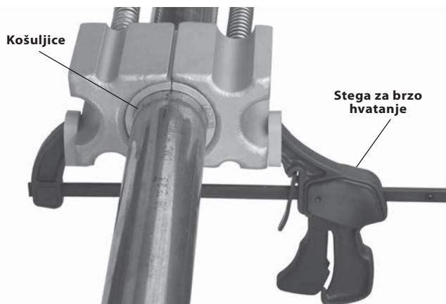
Slika 4 – Pričvršćivanje glava za zamrzavanje stegom za brzo hvatanje
