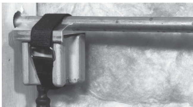
Kuva 7 – Tarranauhalla kiinnitetty päteadapterilla varustettu jäädymispää
