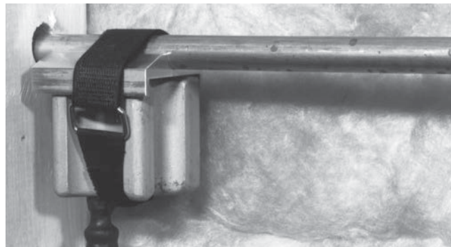
Slika 7 – Glava za zamrzavanje s krajnjim adapterom pričvršćenim čičak-trakom
