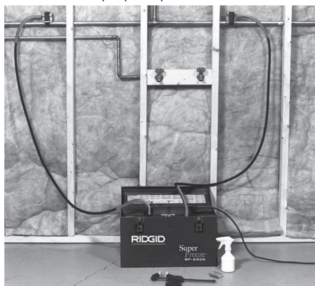
Figura 6 – Congelación de dos tapones
