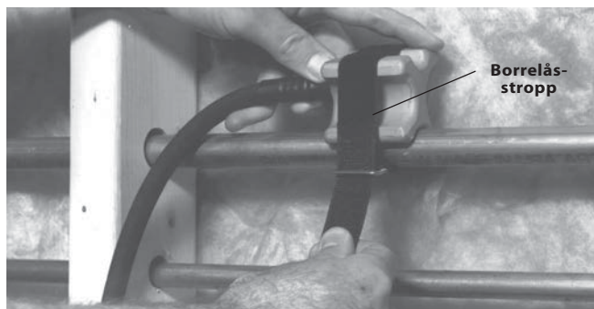
Figur 5 – Bruke frysehode med borrelås-stropp
