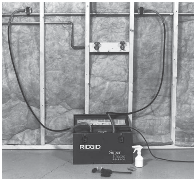
Figur 6 – Dubbel frysning
