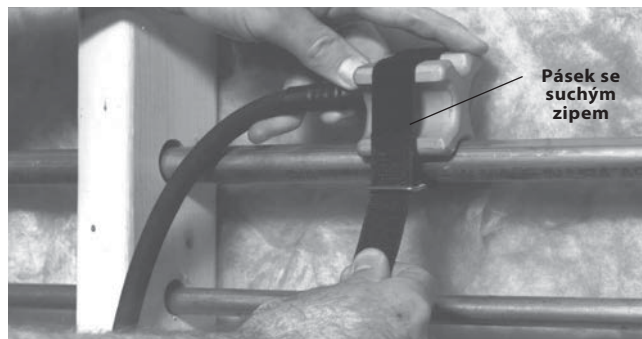
Obrázek 5 – Přichycení mrazicí hlavy pomocí pásku se suchým zipem
