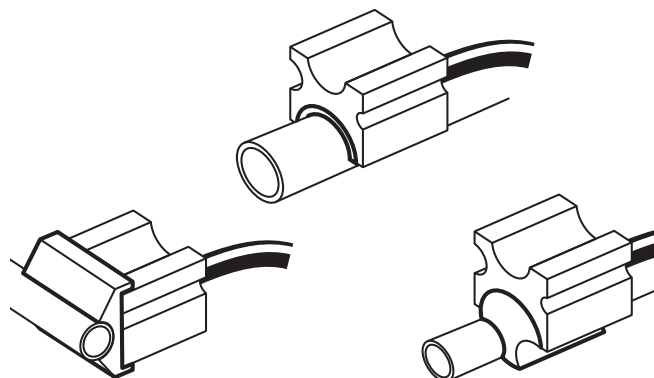
Kuva 8 – Jäädymispäät erilaisilla adaptereilla
