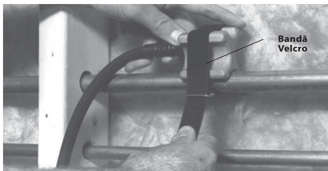
Figura 5 – Aplicarea capetelor de înghețare cu bandă Velcro
