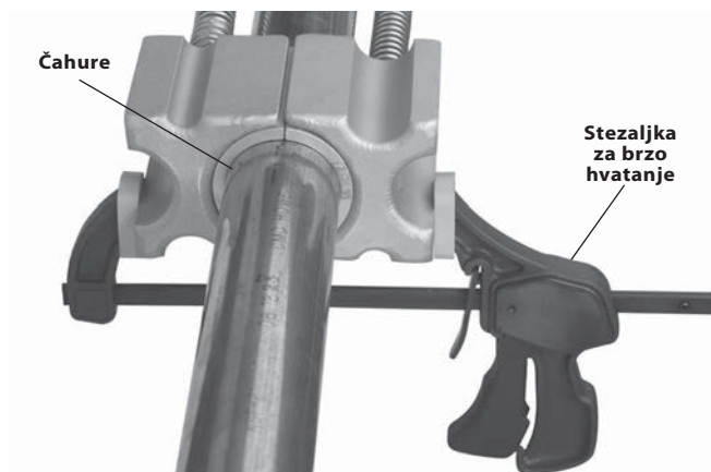
Slika 4 – Spajanje glava za zamrzavanje korištenjem stezaljke za brzo hvatanje
