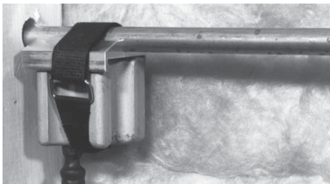
Figuur 7 – Vrieskop met eindadapter bevestigd met klittenband
