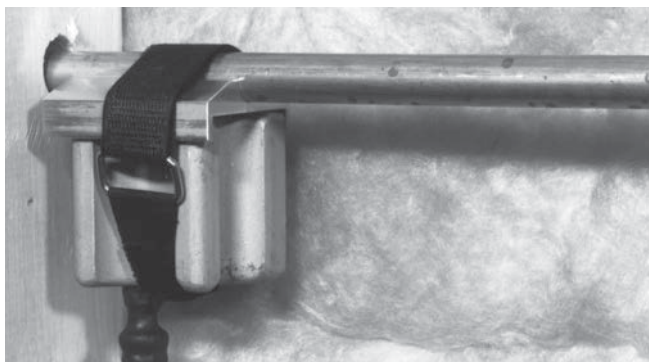
Εικόνα 7 – Ψυκτική κεφαλή με αντάπτορα άκρου στερεωμένο με ιμάντα τύπου βέλκρο
