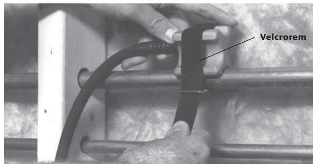
Figur 5 – Fastgørelse af frysehoved med velcrorem
