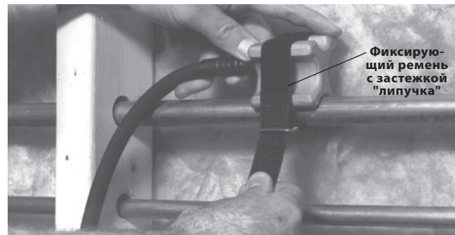
Рис. 5 – Прикрепление замораживающей головки с помощью фиксирующего ремня с застежкой "липучка"
