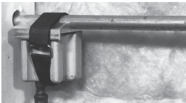
Figura 7 – Testa di congelamento con adattatore a testa con striscia di velcro
