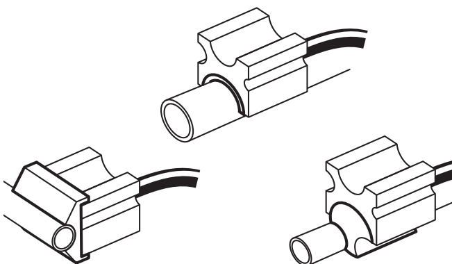
Rys. 8 – Głowice zamrażające z różnymi adapterami
