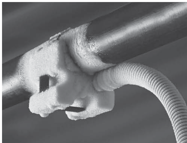
Figur 9 – Fryshuvud fryst vid röret
