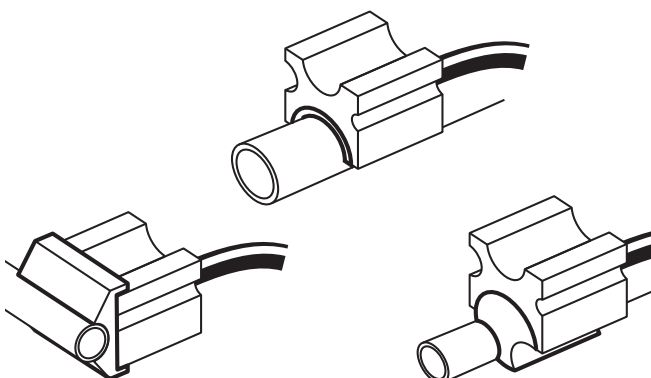
Figuur 8 – Vrieskoppen met verschillende adapters
