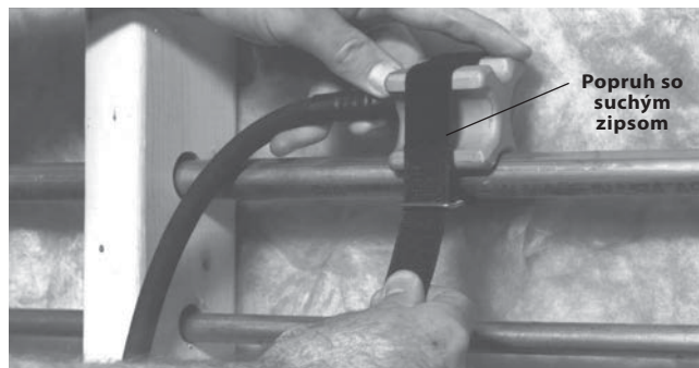
Obrázok 5 – Aplikácia zmrazovacej hlavy s popruhom so suchým zipsom
