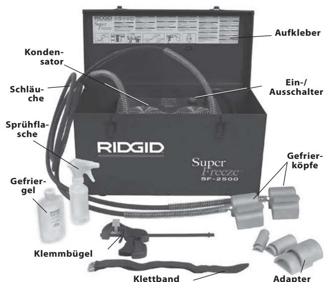
Abbildung 1 – SF-2500 SuperFreeze Gerät
