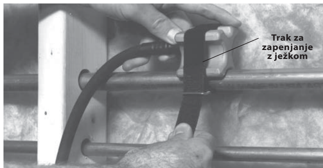
Slika 5 – Namestitev zamrzovalne glave s trakom za zapenjanje z ježkom
