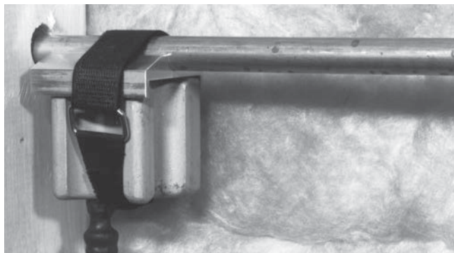
Slika 7 – Glava za zamrzavanje s krajnjim adapterom pričvršćenim Velcro trakom
