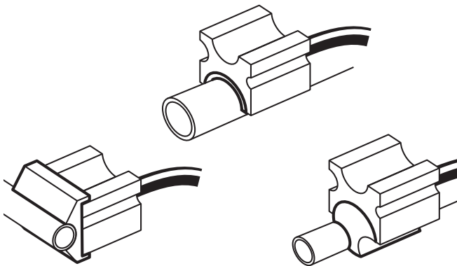
8. ábra – Fagyasztófej a különböző adapterekkel
