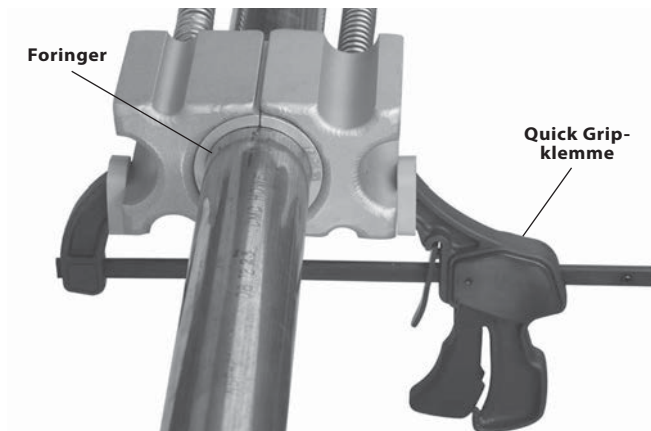
Figur 4 – Feste frysehoder med Quick Grip-klemme
