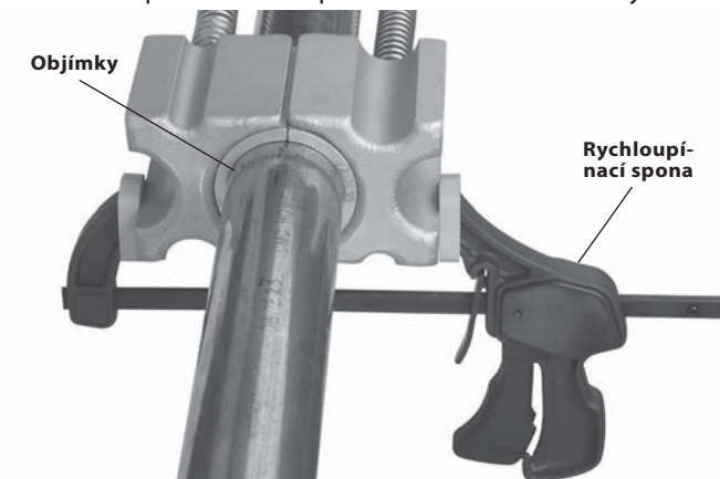
Obrázek 4 – Připojení mrazicích hlav pomocí rychloupínací spony
