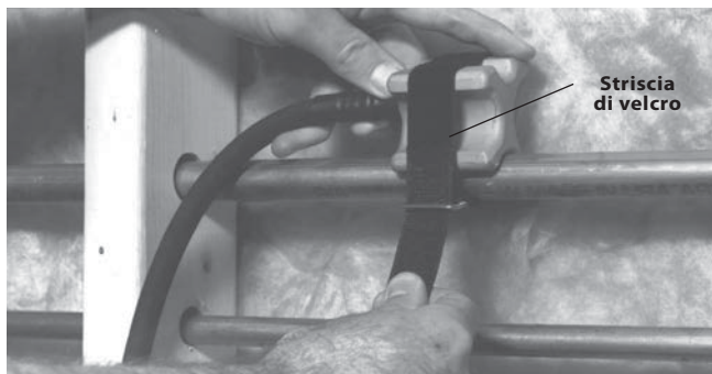
Figura 5 – Applicazione di una testa di congelamento con striscia di velcro
