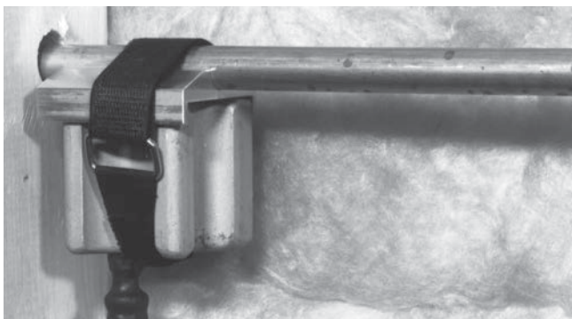
Figur 7 – Frysehoved med endeadapter fastgjort med velcrorem
