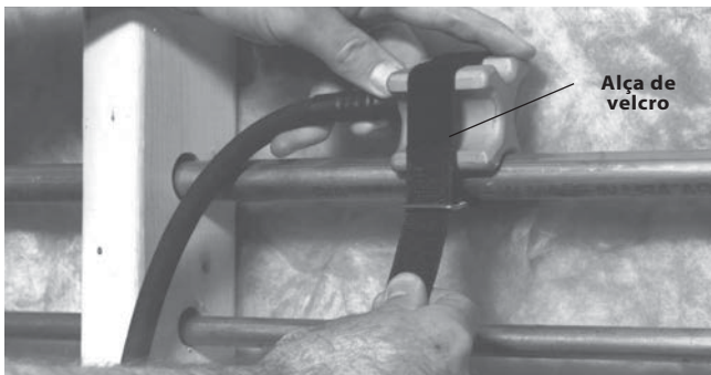
Figura 5 – Aplicar cabeça de congelação com alça de velcro
