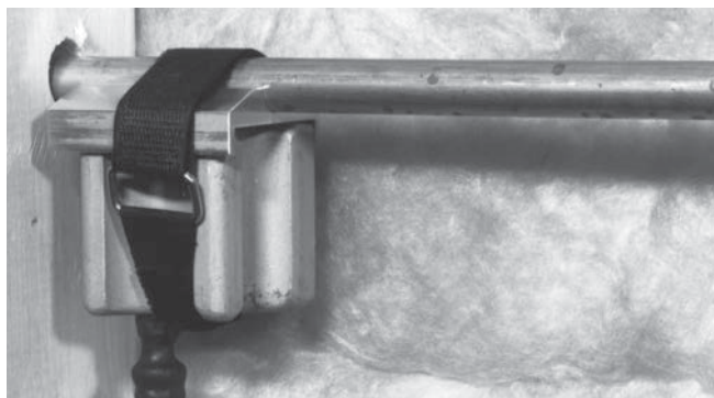
Slika 7 – Zamrzovalna glava s končnim adapterjem pritrjena s trakom za zapenjanje z ježkom
