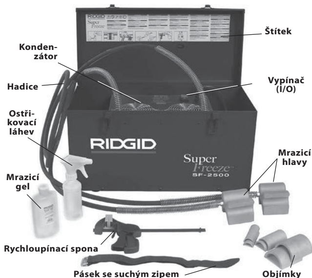
Obrázek 1 – Jednotka na zmrazování trubek SF-2500
