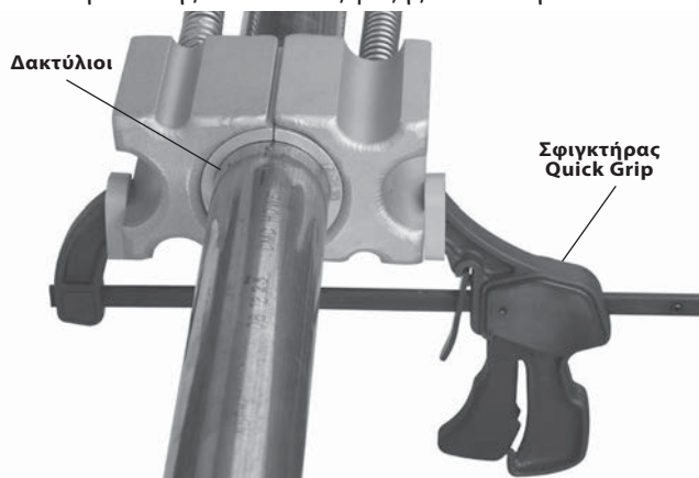
Εικόνα 4 – Τοποθέτηση ψυκτικών κεφαλών με σφιγκτήρα Quick Grip
