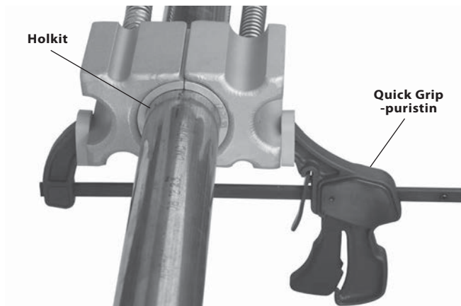
Kuva 4 – Jäädytyspäiden kiinnitys Quick Grip -puristimella
