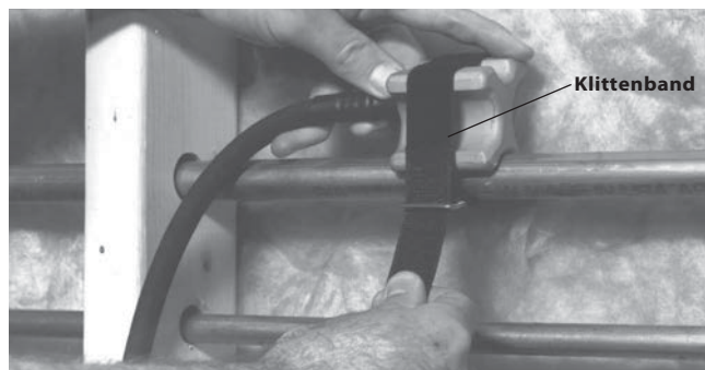
Figuur 5 – Vrieskop bevestigen met klittenband
