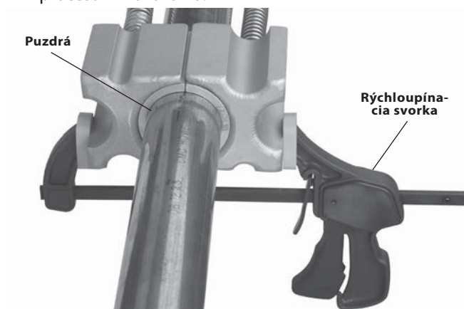
Obrázok 4 – Pripevnenie zmrazovacích hláv pomocou rýchloupínacej svorky
