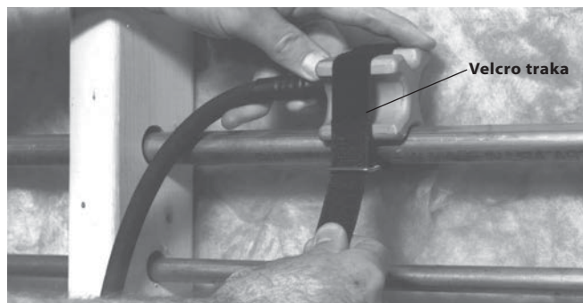
Slika 5 – Primjena glave za zamrzavanje s Velcro trakom
