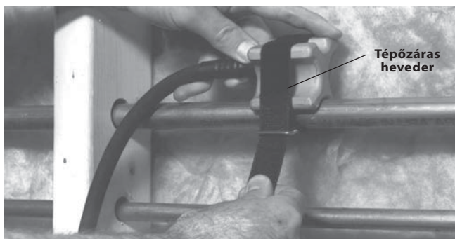
5. ábra – Fagyasztófej a tépőzáras hevederrel
