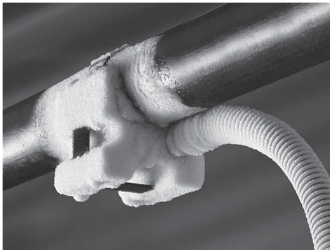
Figure 9 – Tête de congélation et tuyau gelés
