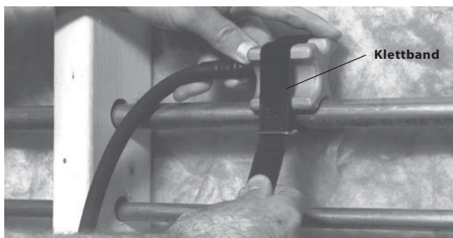
Abbildung 5 – Anbringen des Gefrierkopfs mit Klettband
