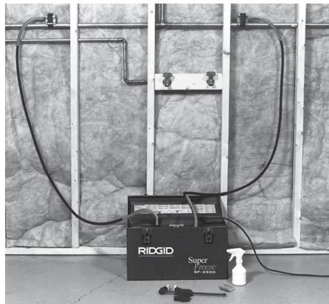
Figure 6 – Création de deux bouchons de glace
