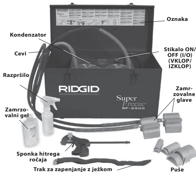
Slika 1 – Enota SF-2500 SuperFreeze
