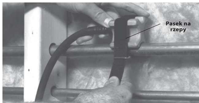
Rys. 5 – Mocowanie głowicy zamrażającej za pomocą paska na rzepy
