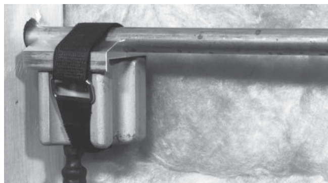
7. ábra – Fagyasztófej a különböző adapterekkel
