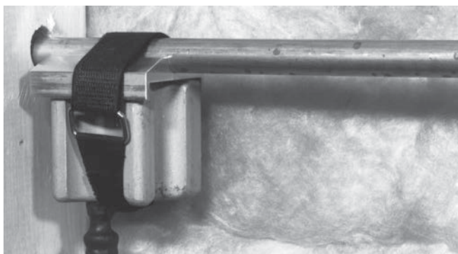
Figura 7 – Cabeça de congelação com adaptador de extremidade fixo com alça de velcro
