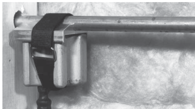
Рис. 7 – Замораживающая головка с концевым переходником, прикрепленная с помощью фиксирующего ремня с застежкой "липучка"
