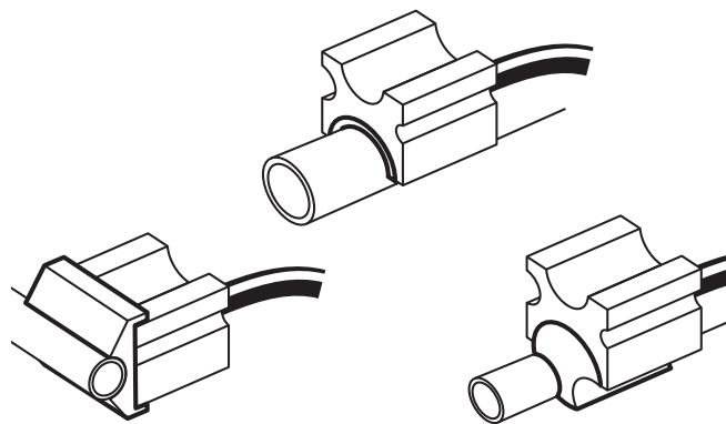
Slika 8 – Zamrzovalne glave z različnimi adapterji
