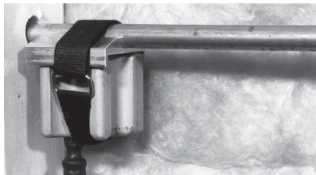
Figure 7 – Tête de congélation équipée d'un adaptateur d'embout et maintenue par une bande Velcro
