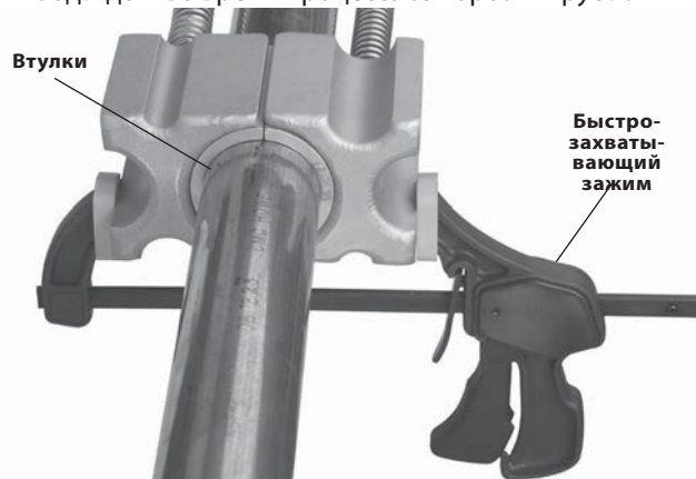
Рис. 4 – Прикрепление замораживающих головок с помощью быстрозахватывающего зажима
