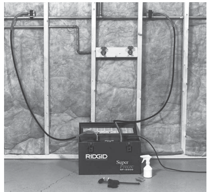
Figura 6 – Aplicação de tampão com duas congelações
