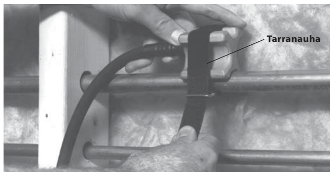
Kuva 5 – Jäädytyspäiden kiinnitys tarranauhalla
