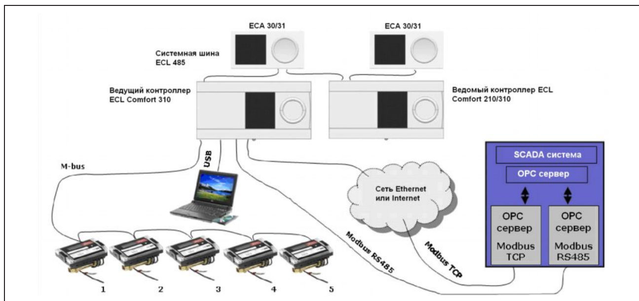
Рис. 2-1: Коммуникационные возможности семейства контроллеров ECL 210/310.
