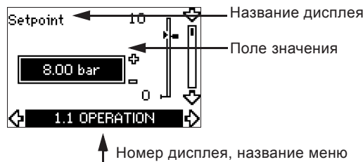
Рис. 47 Пример дисплея в меню пользователя
