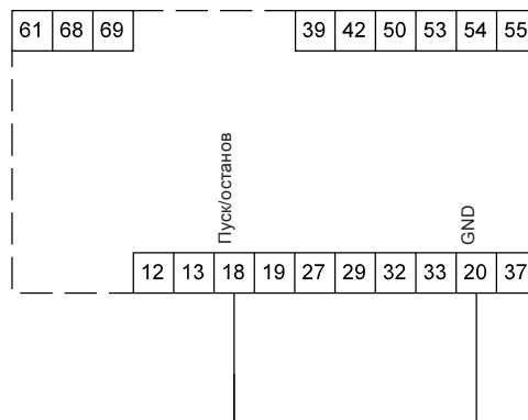
Рис. 22 Минимально необходимые соединения, сигнальные клеммы
