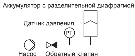
Рис. 50 Расположение обратного клапана и датчика давления в системе с избыточным давлением на входе
