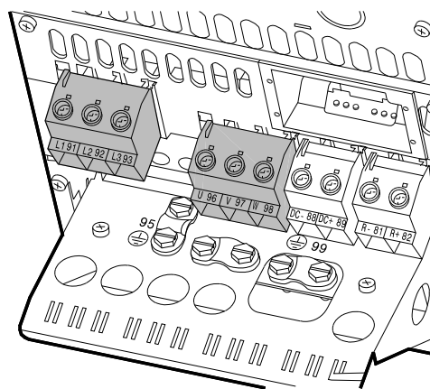
Рис. 17 Подключение питания и двигателя, корпус В4
