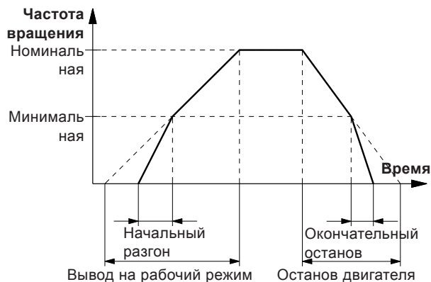
Рис. 53 Вывод на рабочий режим и останов двигателя, экран 3.24
