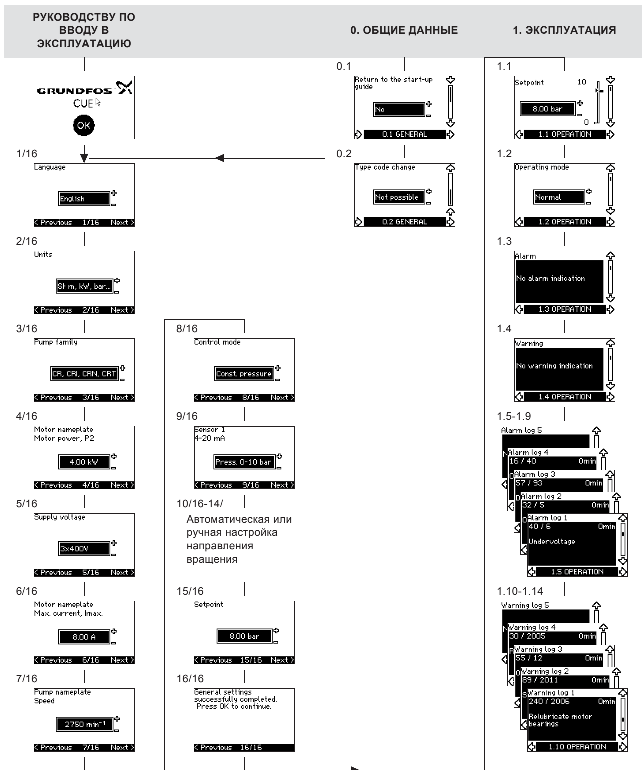
Рис. 44 Обзор меню
