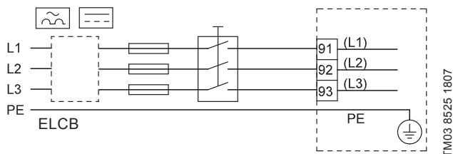
Рис. 5 Пример подключения трехфазного питания устройства CUE с сетевым выключателем, дублирующими предохранителями и дополнительной защитой.
