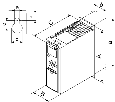
Рис. 57 Корпусы A2 и A3
