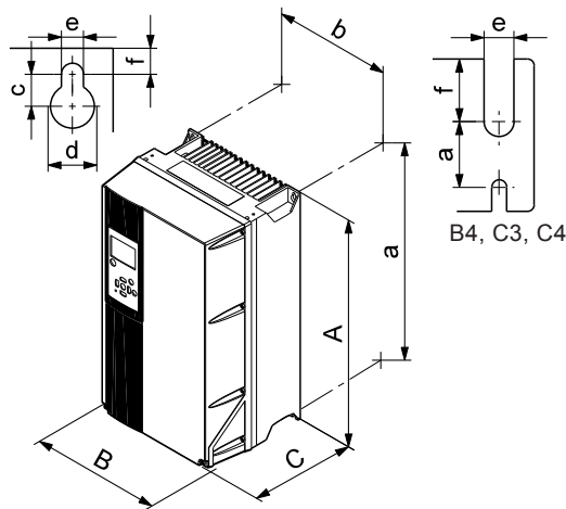
Рис. 58 Корпусы A5, B1, B2, B3, B4, C1, C2, C3 и C4
