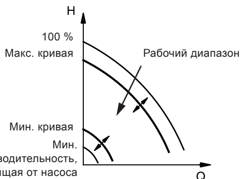
Рис. 52 Настройка минимальной и максимальной кривых в процентах от максимальной производительности
