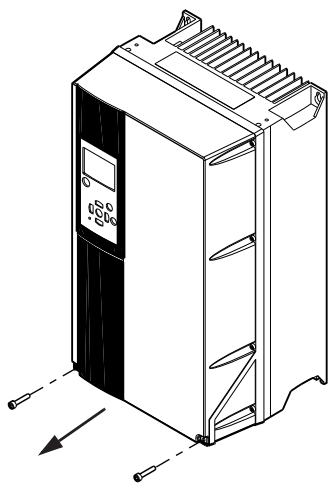
Рис. 24 Доступ к сигнальным клеммам, корпуса A5, B1, B2, B3, B4, C1, C2, C3 и C4
