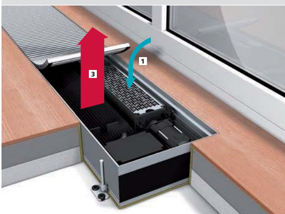
Системный конвектор с тангенциальным вентилятором – QSK
