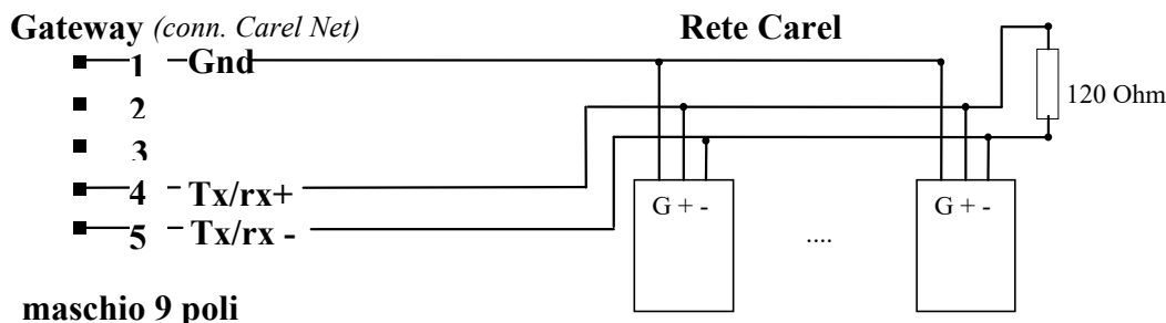
Fig. 7.1.1.1 - Connessione in 485
