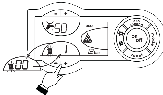
рис. 19 - Режим TEST (мощность отопления = 100%)
