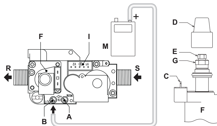
рис. 20 - Газовый клапан
