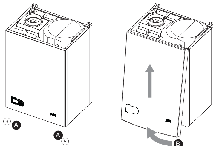
рис. 21 - Демонтаж кожуха
