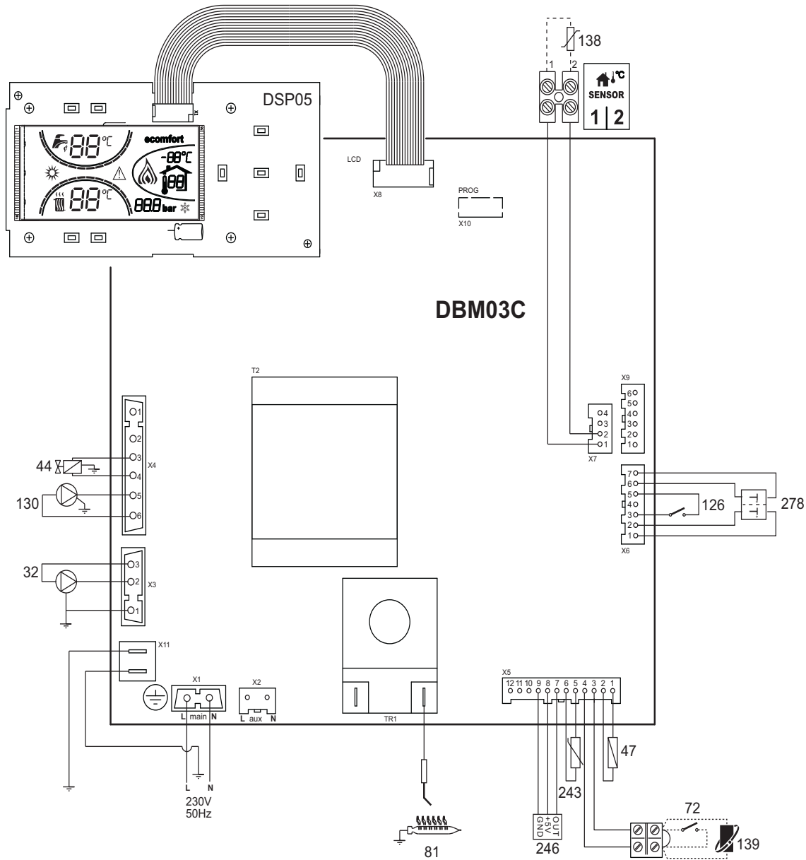
рис. 25 - Электрическая схема
