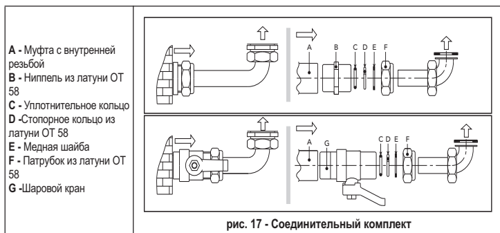
рис. 17 - Соединительный комплект
