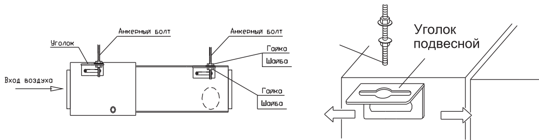
Рис. 10.26 — Установка блока
