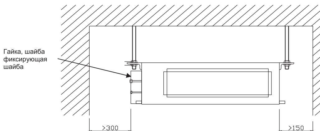
Рис. 10.24 — Размещение блока
