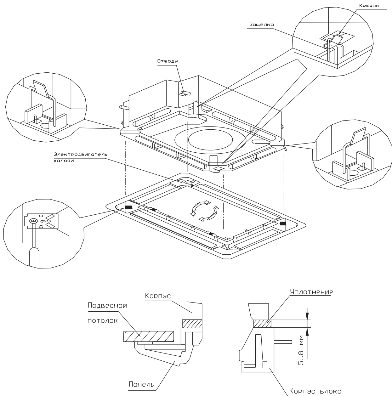
Рис. 10.20 — Установка панели
