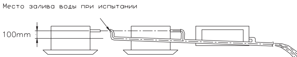
Рис. 12.1 — Проведение гидравлических испытаний
