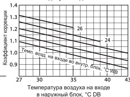
Холодопроизводительность
