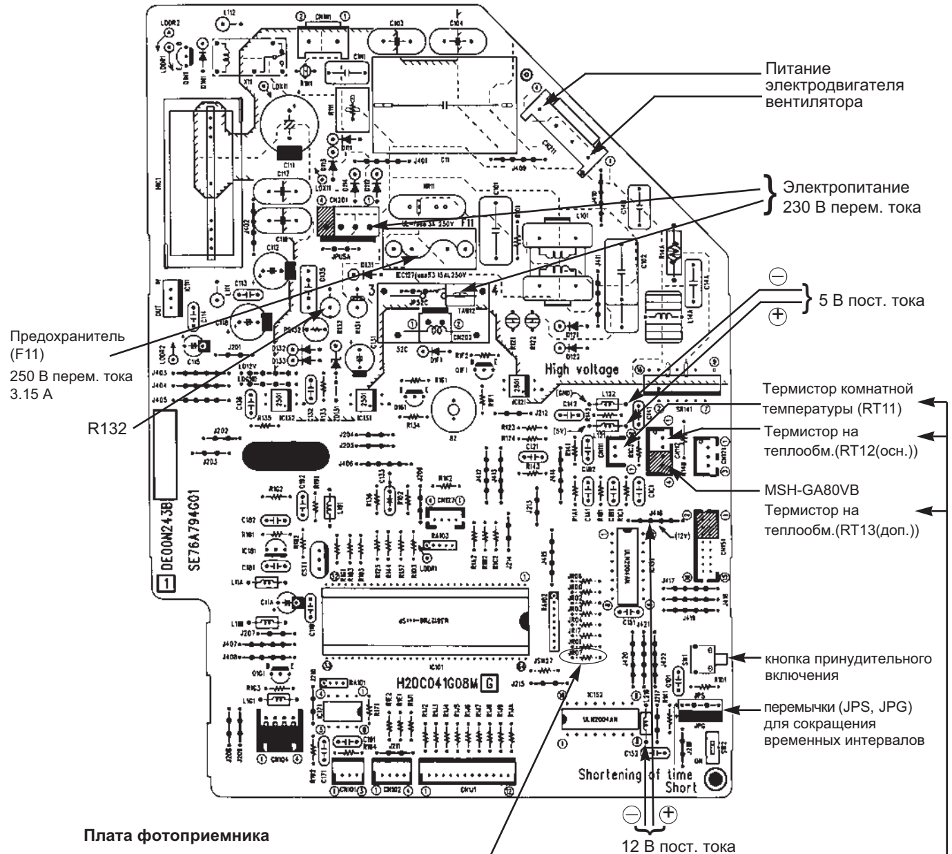
Термистор на теплообм.(RT12(осн.), RT13(доп.)) Термистор комнатной температуры (RT11)
