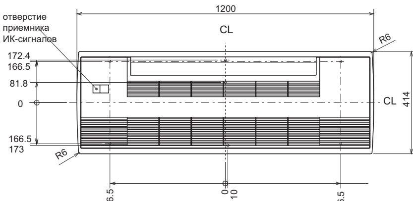
Вид сверху
