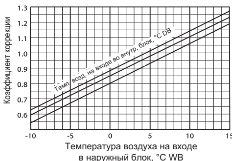
Теплопроизводительность
