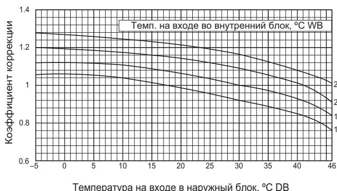
Рис. 1. Холодопроизводительность
