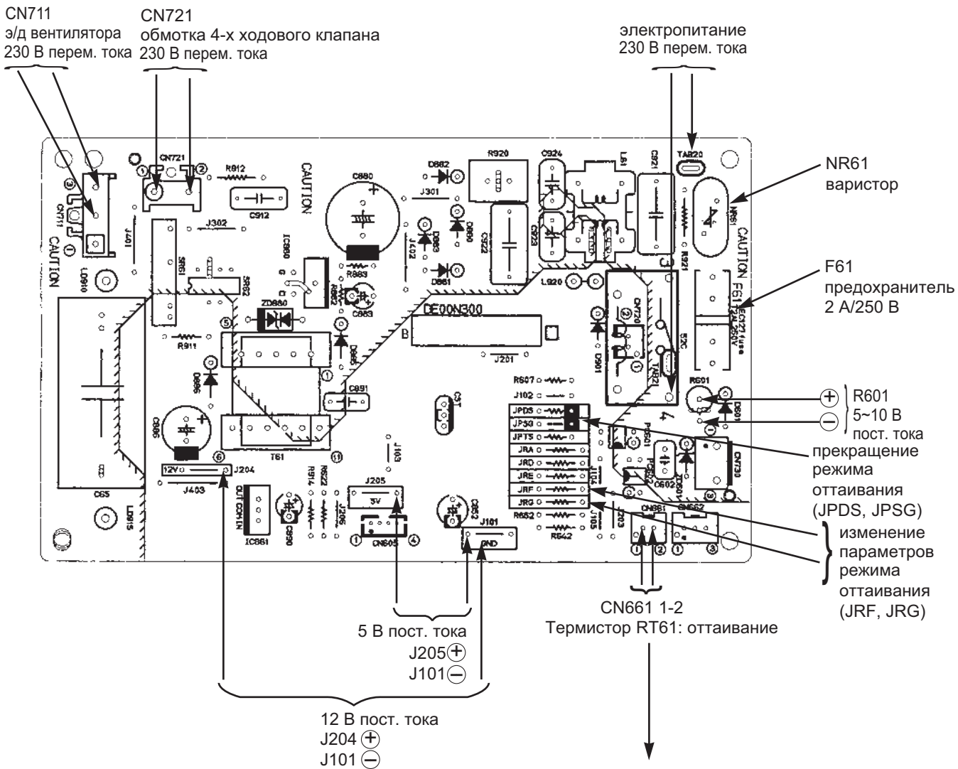
Термистор RT61: оттаивание
