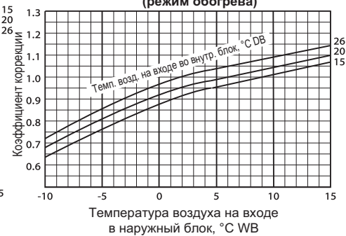
Потребляемая мощность (режим обогрева)
