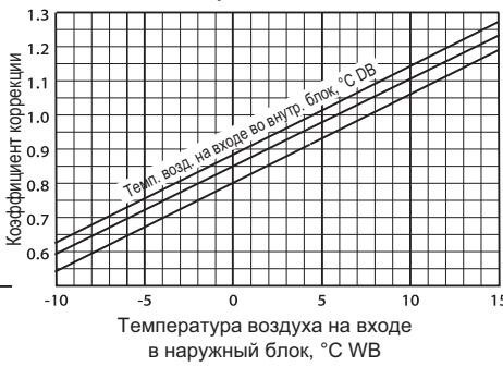
Теплопроизводительность
