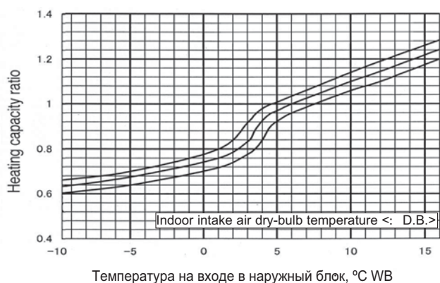
Рис. 3. Теплопроизводительность
