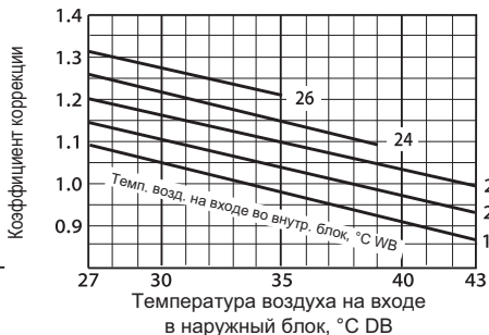
Холодопроизводительность
