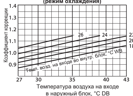
Потребляемая мощность (режим охлаждения)
