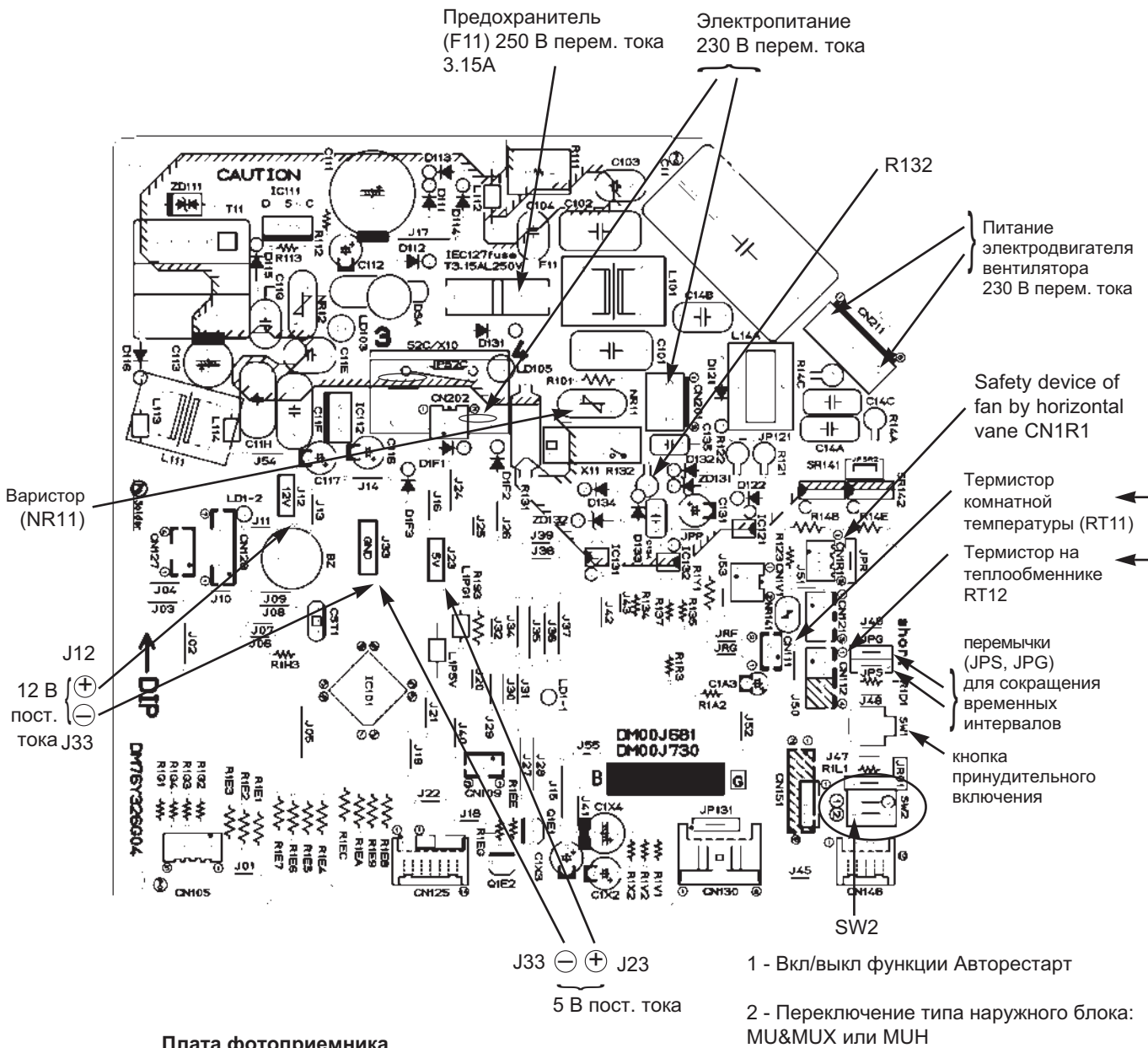
Термистор на теплообменнике RT12 Термистор комнатной температуры (RT11)
