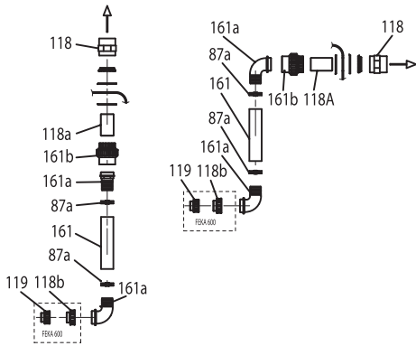
Вертикальный напорный патрубок Горизонтальный напорный патрубок
