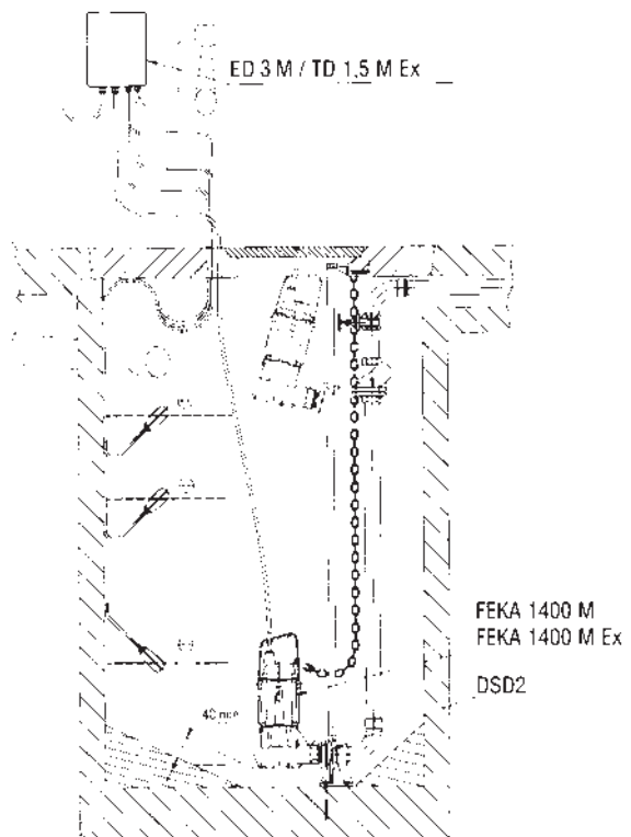
Схема стационарной установки с одним насосом FEKA 1400 M или FEKA 1400 M-Ex укомплектованным подъемным устройством DSD2, шкафом управления и защиты ED 3 M или TD 1.5 M Ex, двумя управляющими поплавками уровня (минимальный и максимальный) и одним аварийным поплавком
