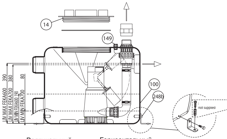
Вертикальный напорный патрубок Горизонтальный напорный патрубок
