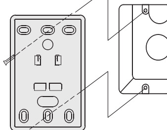
термостат кронштейн
