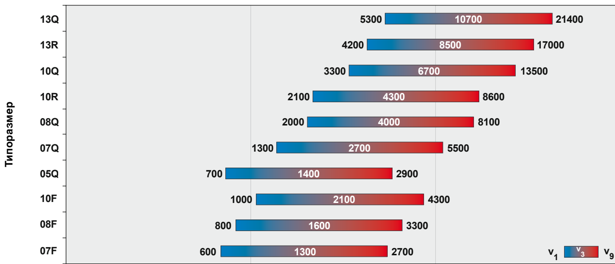
Производительность (м³/ч)
