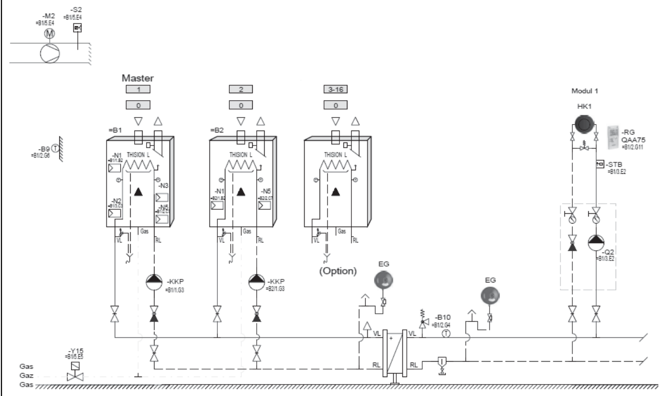
1-В-С-Е: 1 отопительный контур + каскад через пластинчатый теплообменник
