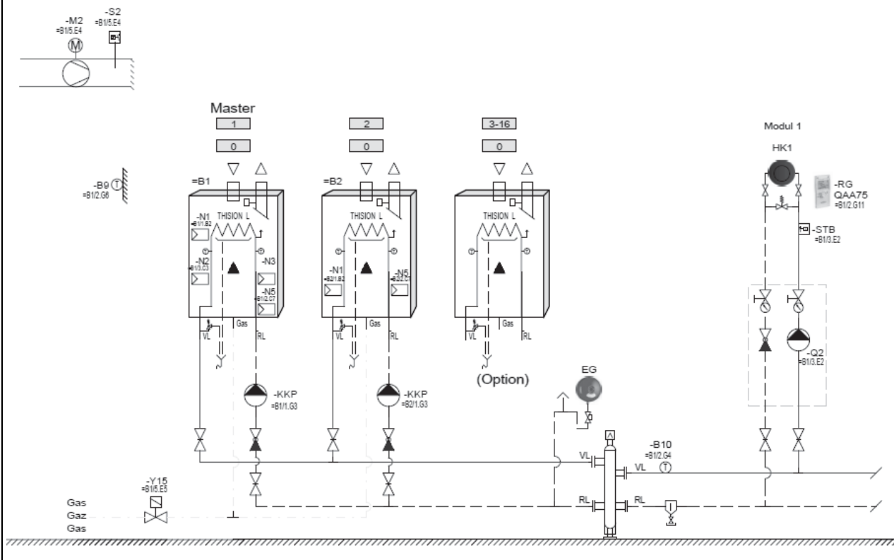
1-А-С-Е: 1 отопительный контур + каскад через гидравлический разделитель
