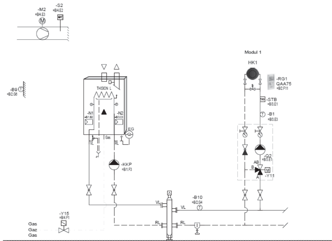
2-A-C: 1 смешанный отопительный контур + гидравлический разделитель
