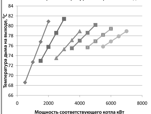
График температуры выхода дыма при температуре возврата от 60° до 80°С
