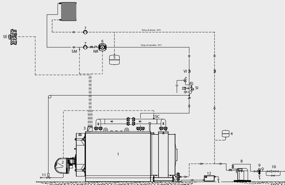
Схема установки для котла GREENOX BT COND : 1 прямая зона, 1 генератор
