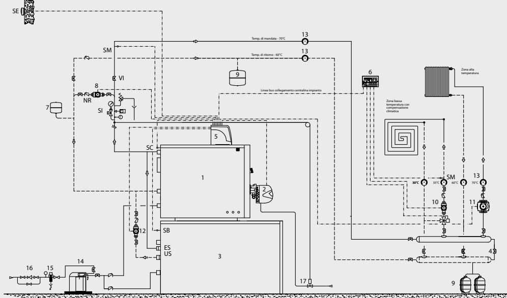
Схема установки для котлов модели BLUNOX.e B : 1 прямая зона, 1 смешанная зона, 1 генератор, 1 встроенный бойлер
