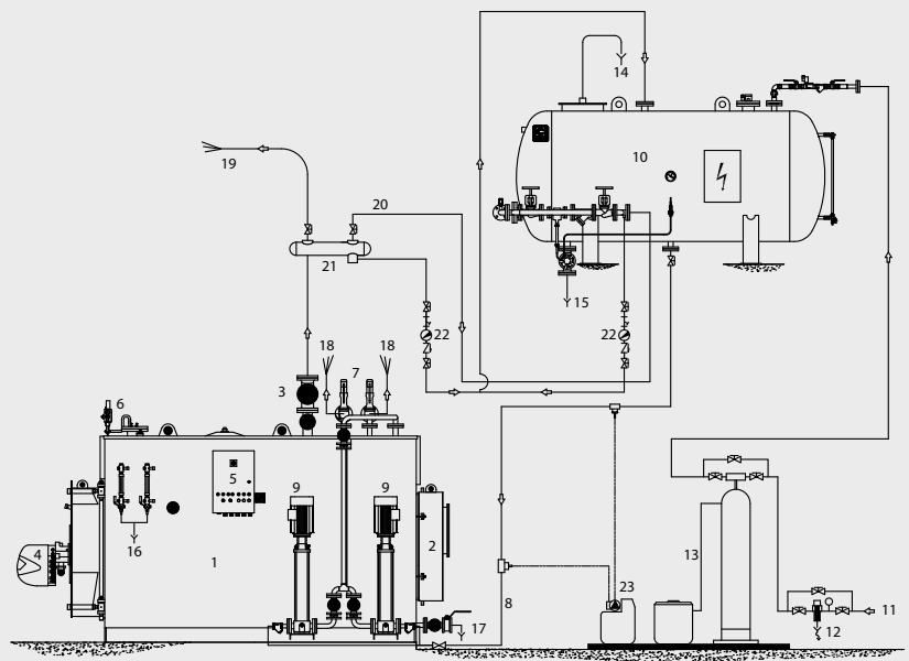
Схема системы без рекуперации конденсата для парогенераторов моделей SIXEN, BX, FX, GX и GXС
