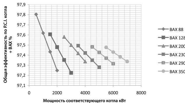
График КПД генератора и BAX при температуре возврата от 60° до 80°С
