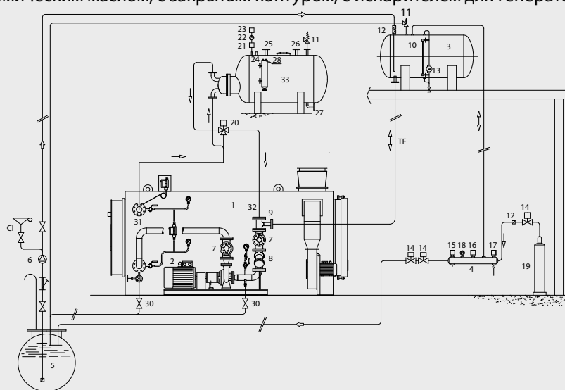
Схема системы с диатермическим маслом, с закрытым контуром, с испарителем для генераторов модели OPX REC
