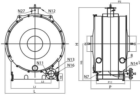
МОД. 88 ÷ 128
