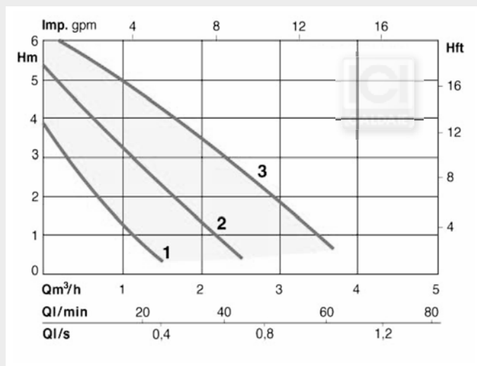
ГРАФИК ОСТАТОЧНОГО НАПОРА
