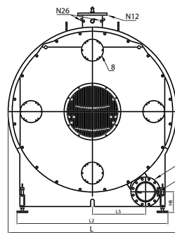
МОД. 200 ÷ 350
