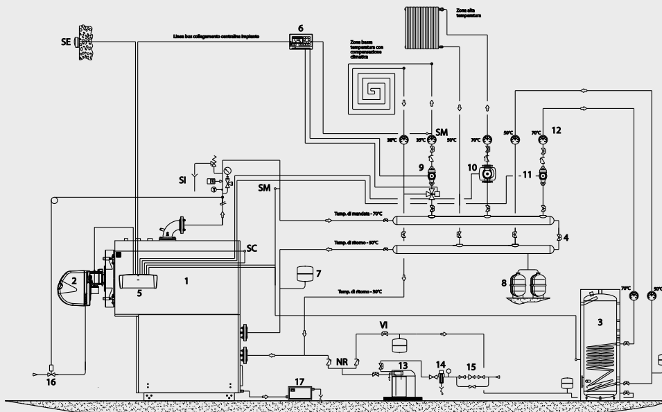
Схема установки для котлов MONOLITE JB, MONOLITE GT, CODEX и STELT : 1 прямая зона, 1 смешанная зона, 1 генератор, 1 бойлер
