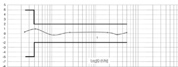
Типичная кривая погрешности
