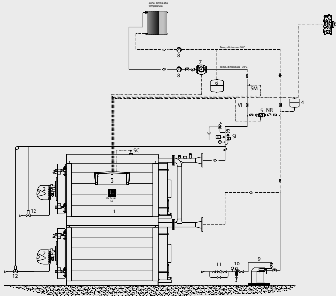
Схема установки для котлов моделей REX DUAL и REX DUAL F : 1 прямая зона, 2 генератора каскадной установки
