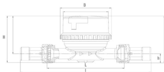
Габариты
