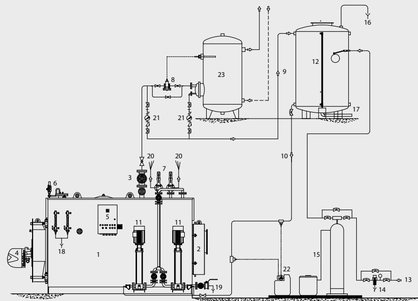
Схема системы с рекуперацией конденсата для парогенераторов моделей SIXEN, BX, FX, GX и GXС
