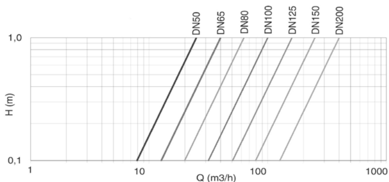
Потери нагрузки
