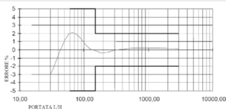
Типичная кривая погрешности (75/33/ЕЕС ВОДА ПРИ 30 °C)
