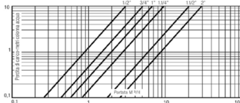
Потери нагрузки
