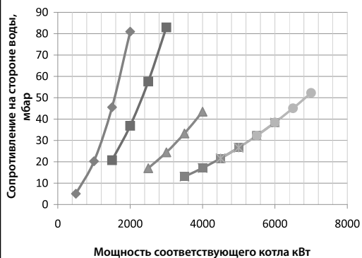
График сопротивления на стороне воды при температуре возврата от 60° до 80°С
