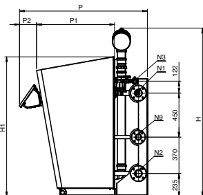
ТВХ ДВОЙНОЙ/ТРОЙНОЙ
