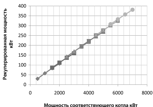
График рекуперированной мощности при температуре возврата от 60° до 80°С
