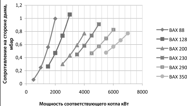
График сопротивления на стороне дыма при температуре возврата от 60° до 80°С
