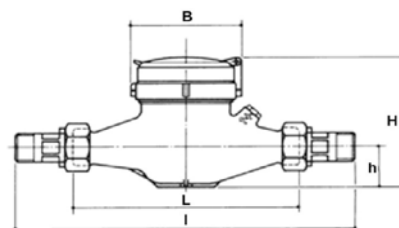
Габариты
