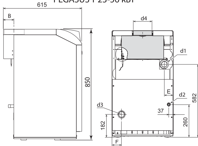
PEGASUS T 23-56 кВт
