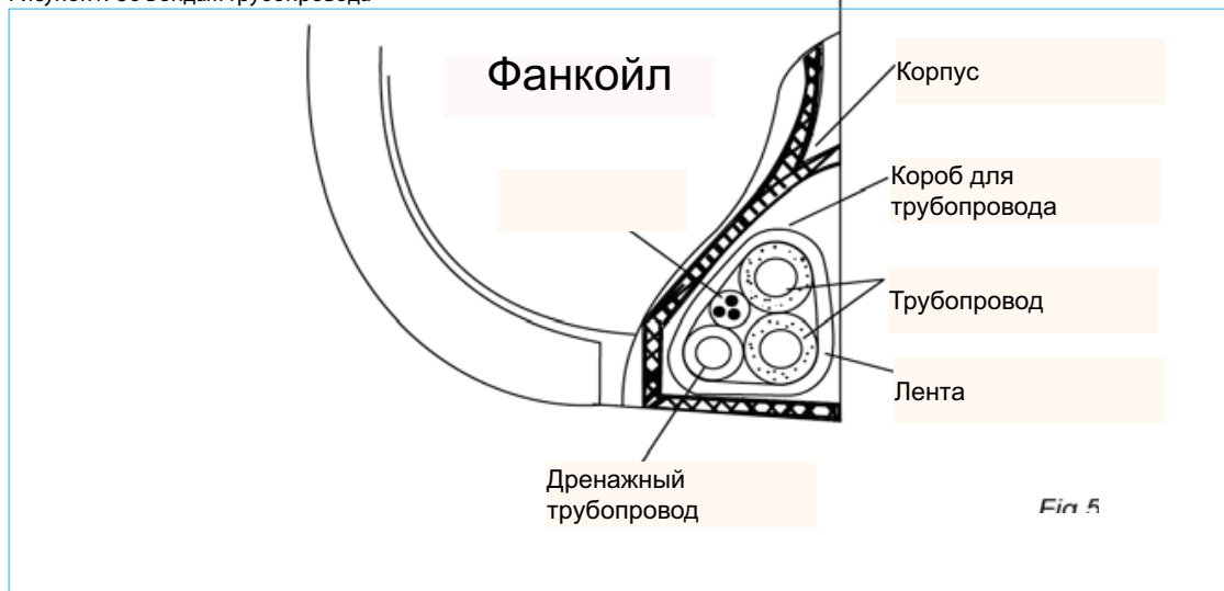
Рисунок №56 Бандаж трубопровода
