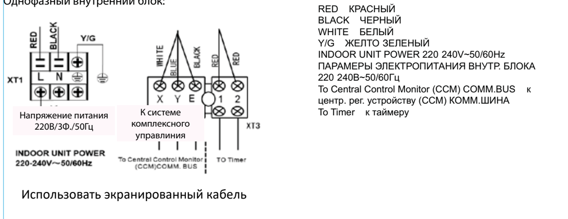
Рисунок №63 Схема клеммной колодки
