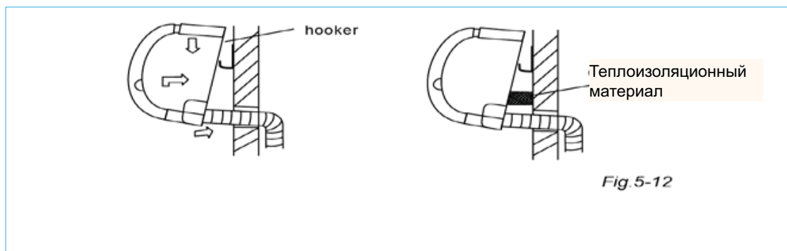
Рисунок №57 Монтаж внутреннего блока
