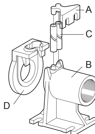
Fig. 7 Piede d'accoppiamento
