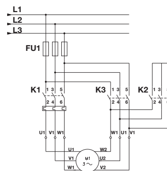
Fig. 11 conexión estrella-triángulo
