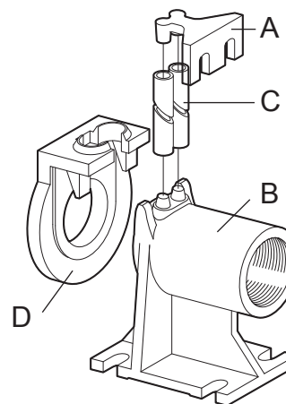
Rys. 7 Nóżka podtrzymująca
