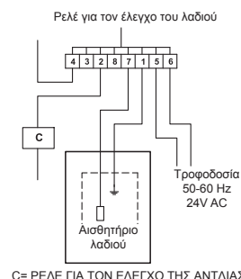
Εικ. 14 Σύνδεση αισθητηρίου στάθμης!
