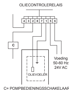
Afb. 11 Aansluiting niveuvoeler
