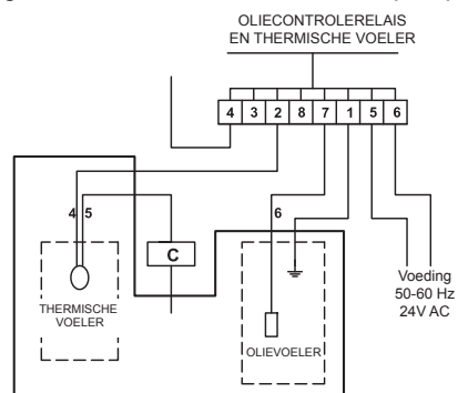
Afb. 10 Aansluiting niveuvoeler
