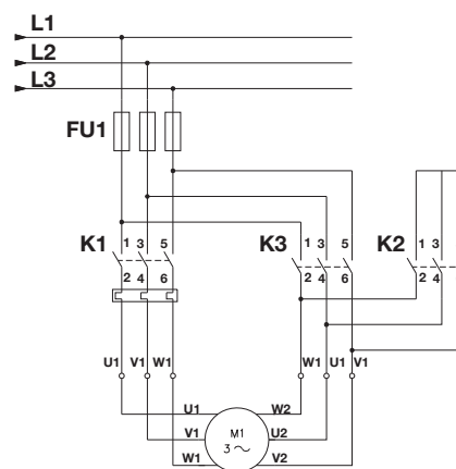
Схема 11 Соединения со звезды на треугольник
