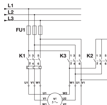
Afb. 11 Ster-driehoekaansluitingen
