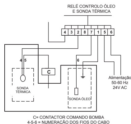
Fig. 13 Ligação da sonda térmica
