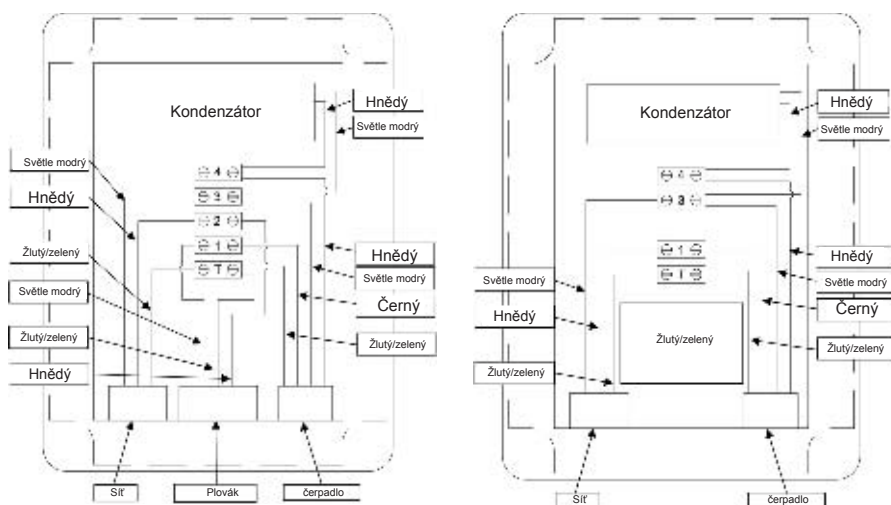
Obr. 8 Schémata elektrického připojení jednofázového čerpas plovákem a bez plováku.
