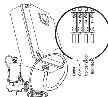
Fig. 9 Quadro eléctrico para bombas de baixa tensão
