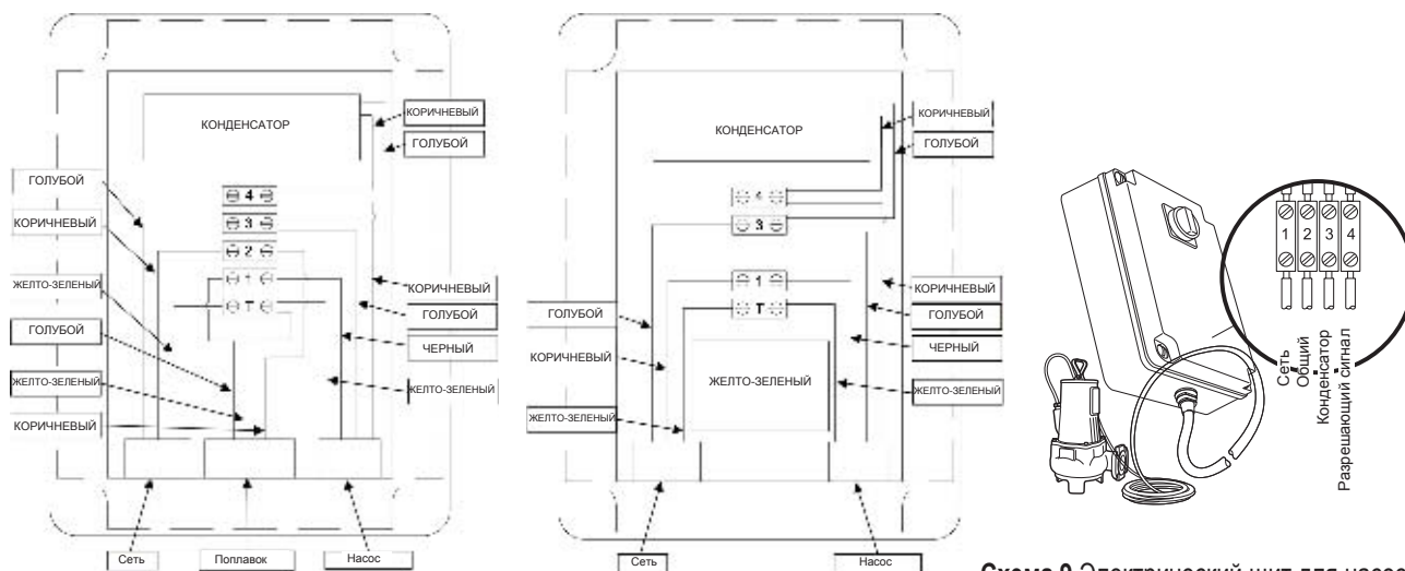
Схема 8 Схемы электрического подключения монофазного насоса с поплавком и без него
