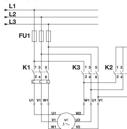
Fig. 11 Ligações estrela triângulo
