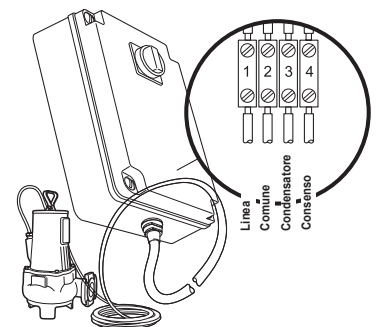
Fig. 9 Esquema de conexión eléctrica para las electrobombas baja tensión
