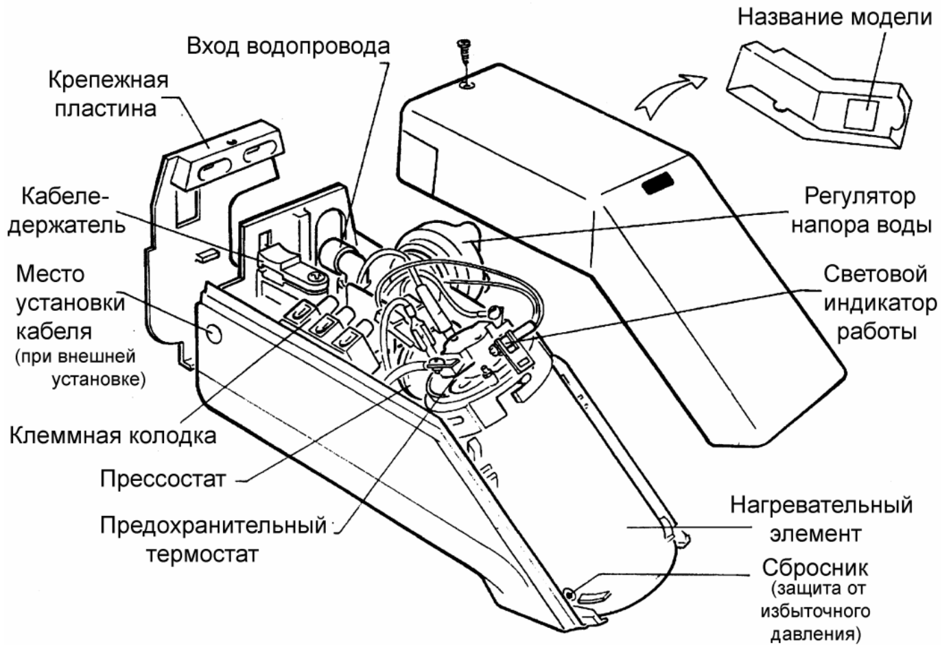
Рис. 1.0 Устройство водонагревателя
