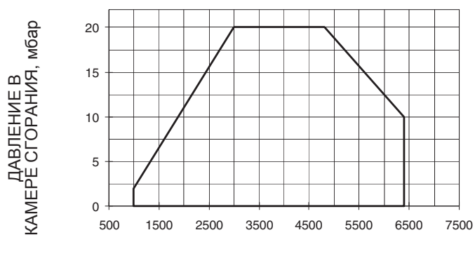
R520A M-....VS.x.50/65/80/100
