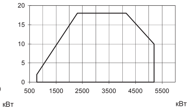
R525A M-....VS.x.50/65/80/100
