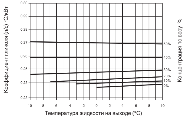
Рис. 6 - Коэффициенты для другой концентрации пропилен гликоля
