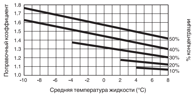
Рис. 8 - Поправочные коэффициенты падения давления для жидкости с пропилен гликолем
