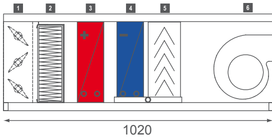
1. Многостворчатый клапан. 2. Воздушный фильтр. 3. Водяной воздушонагреватель. 4. Воздухоохладитель. 5. Каплеотделитель. 6. Вентилятор.
