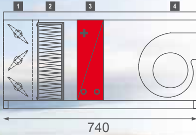
1. Многостворчатый клапан. 2. Воздушный фильтр. 3. Водяной воздушонагреватель. 4. Вентилятор.
