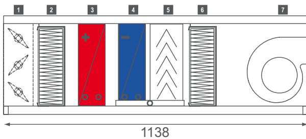
1. Многостворчатый клапан. 2. Воздушный фильтр F5. 3. Водяной воздушонагреватель. 4. Воздухоохладитель. 5. Каплеотделитель. 6. Воздушный фильтр F7. 7. Вентилятор.
