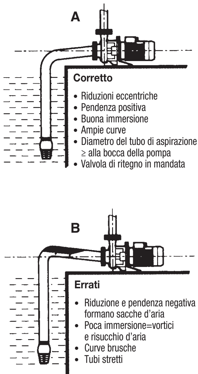
fig. 1 - schema installazione
