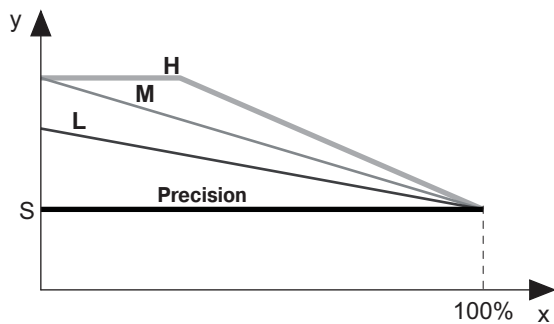
AdaptiveFunction Plus для режима охлаждения
