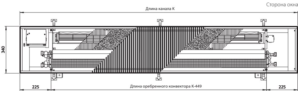
Вид сверху (вид без крышки)
