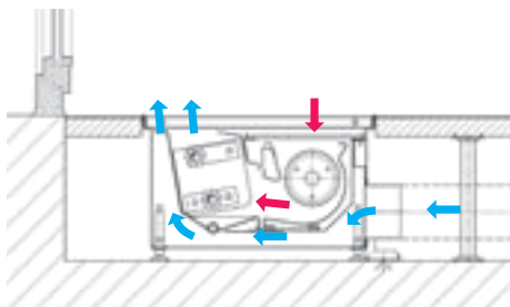
Разрез (пример с роллонной решеткой)
