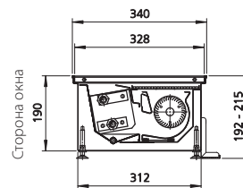
Разрез (пример с рулонной решеткой)
