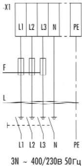
Питание горелки
