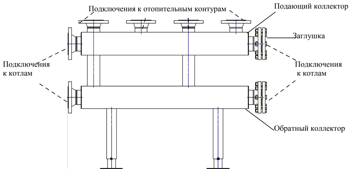
Рис. 3. 2-х контурный коллектор Ду65, Ду80, Ду100, Ду125, Ду150
