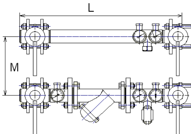
Рис.6. Подключение коллектора
